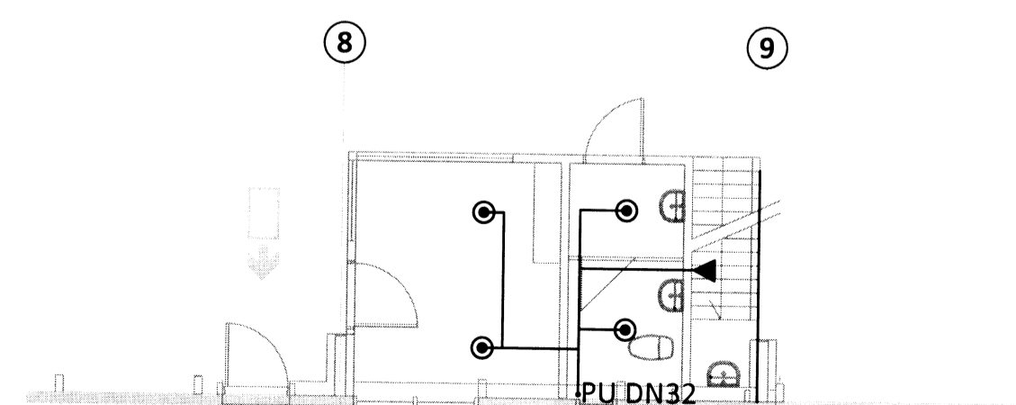
GRUNNMYND 1.HÆÐ M1:100
