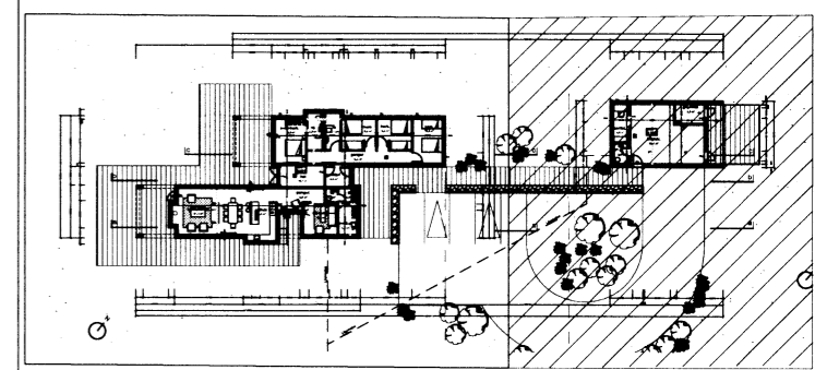
Grunnmynd / yfirlit - Bílskúr/geymsla 1 2
