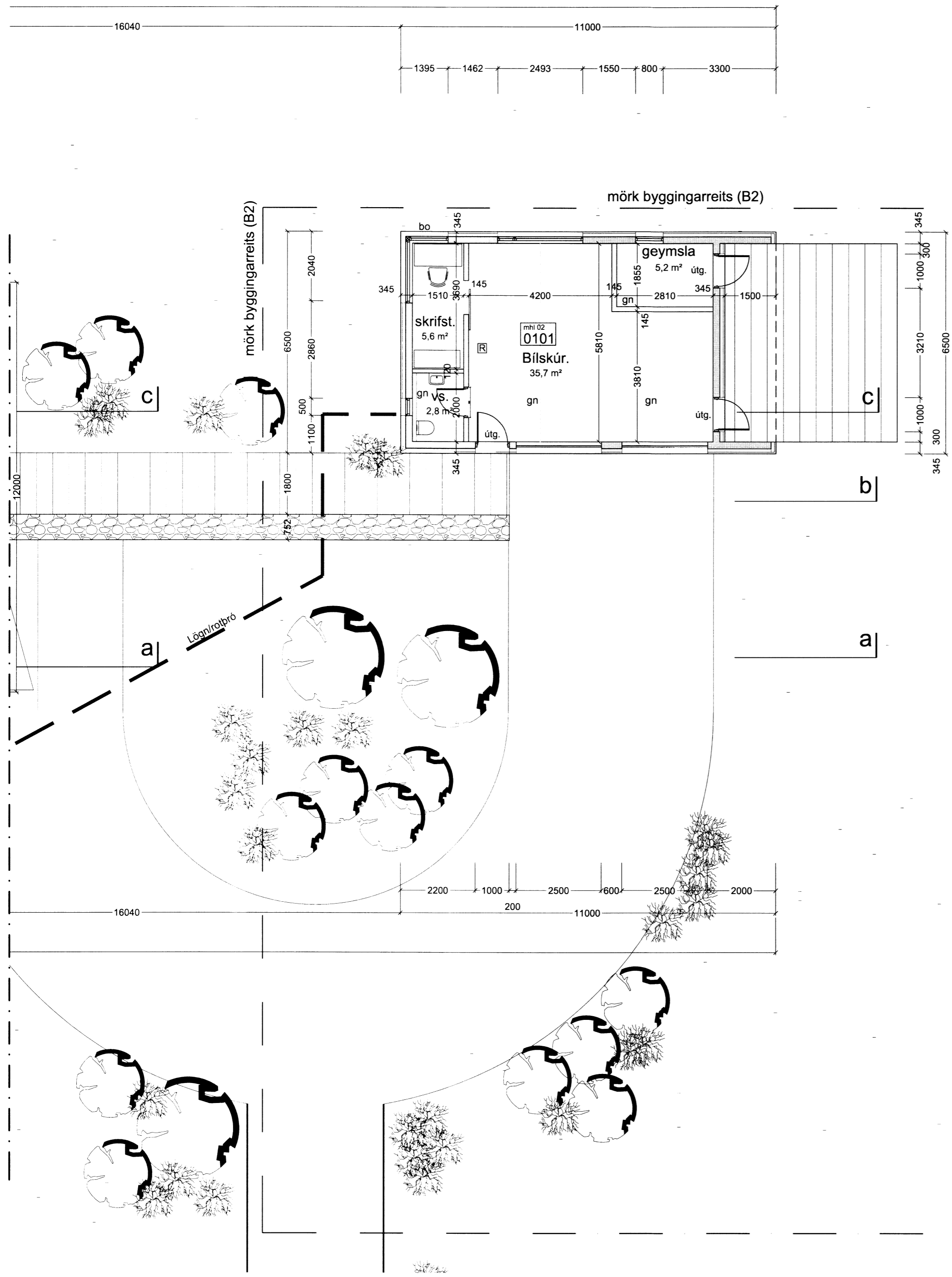
Grunnmynd - 1: 100 (Bílskúr - 2)
