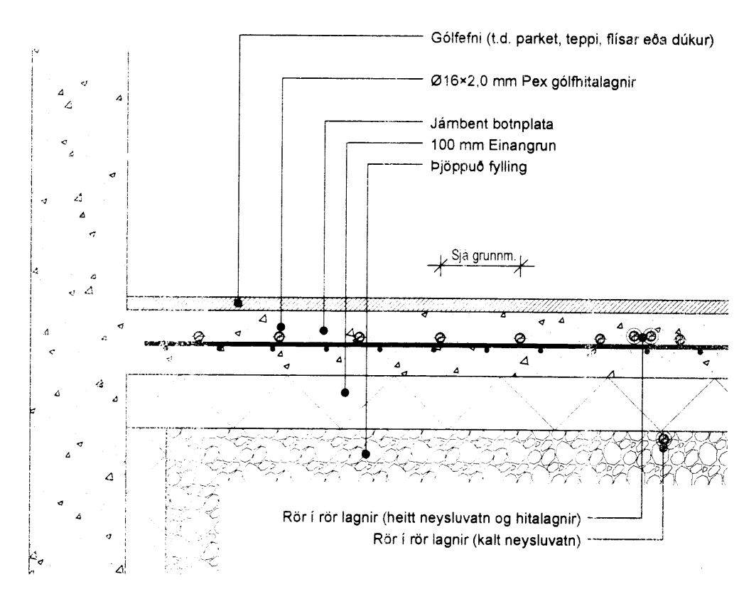
KENNISNIÐ GÖLFHITA 1:10
