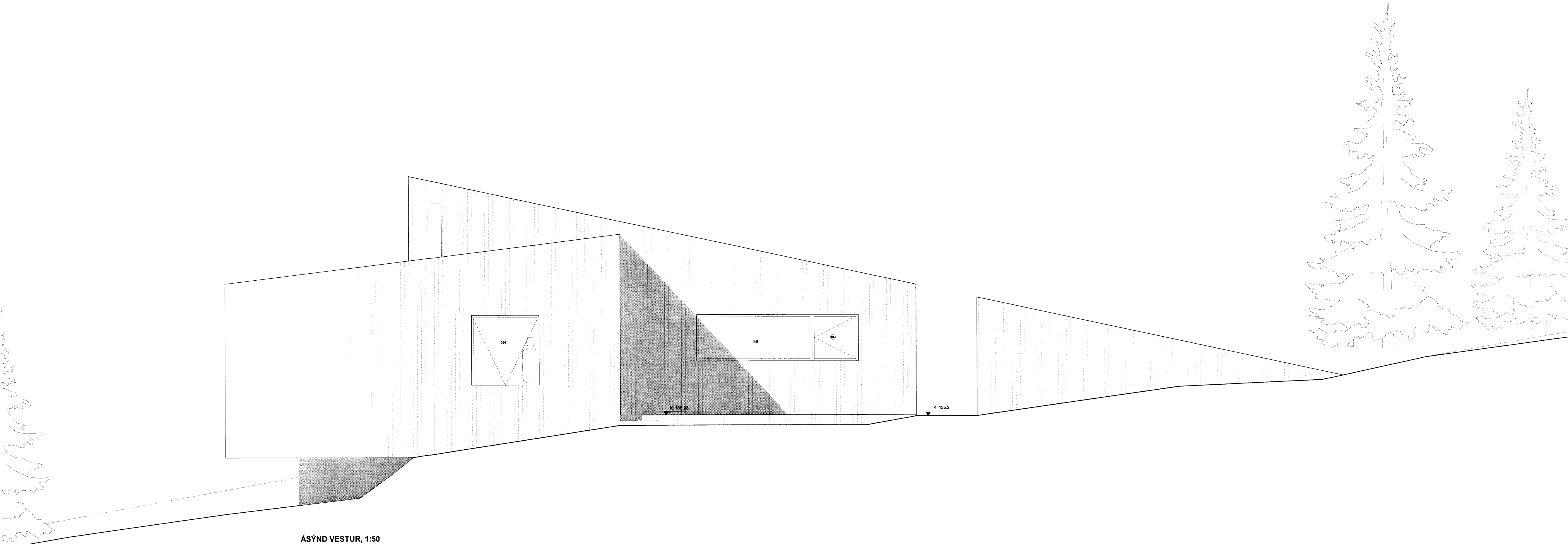
ÁSYND VESTUR, 1:50
