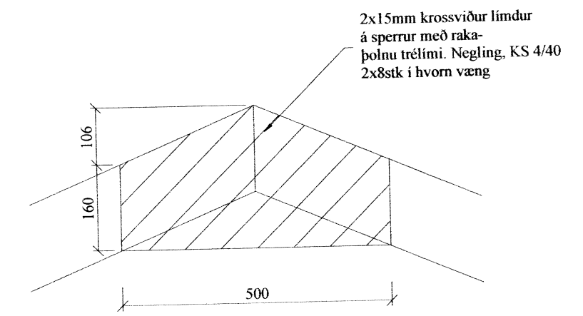
FS3. Samsetning sperra í mæni kvista
