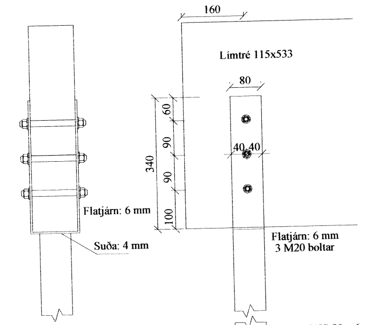
FS9. Stálsúla undir limtré
