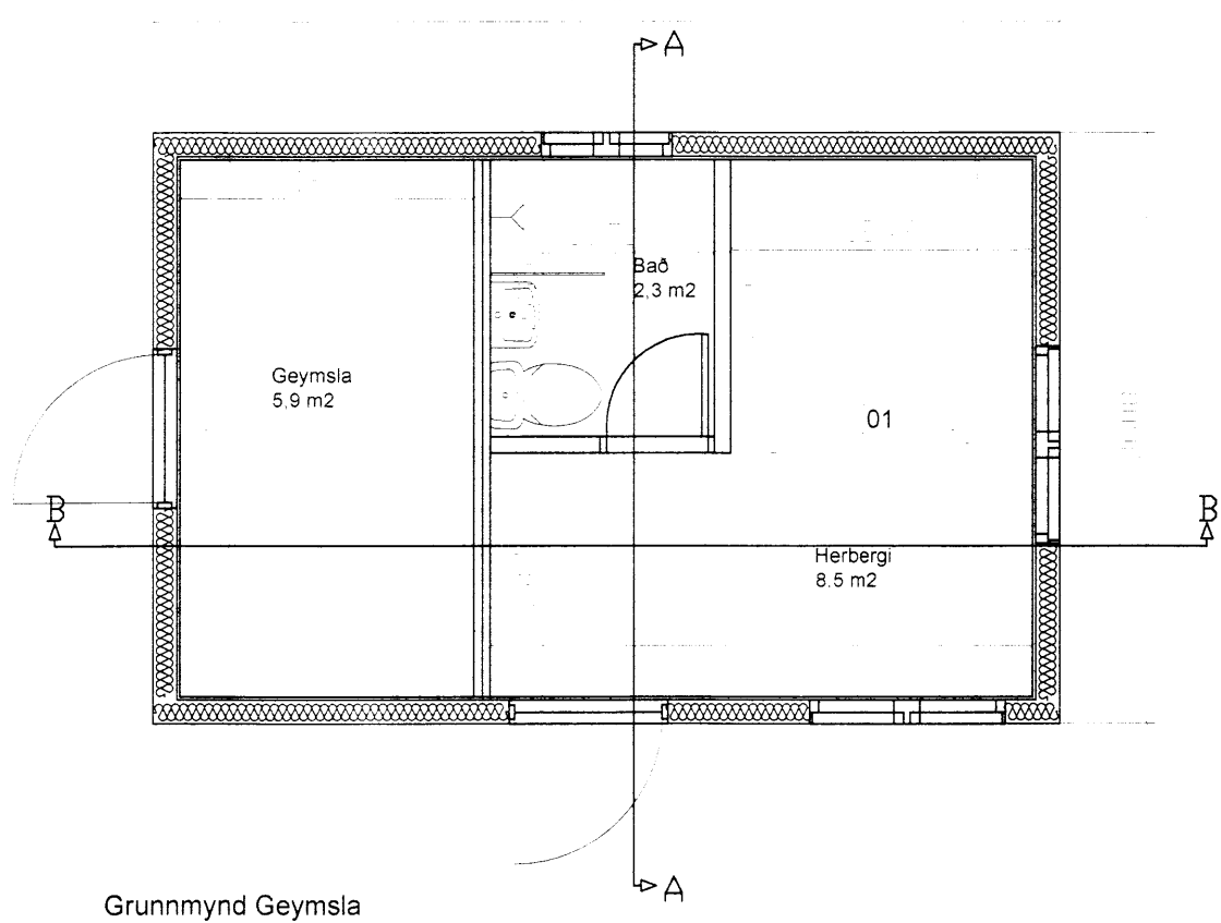
Grunnmynd Geymsla
