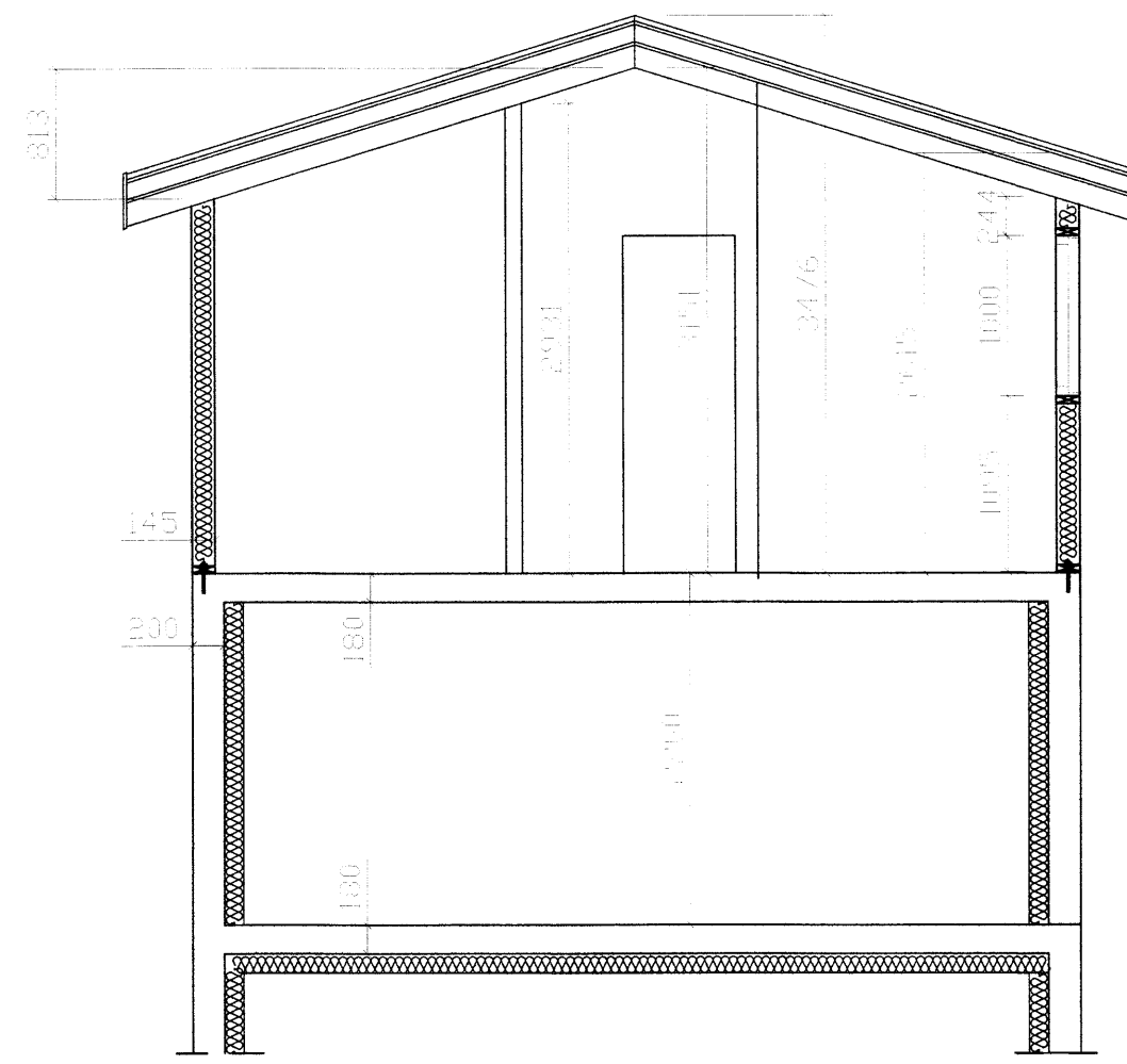
Snið B-B
