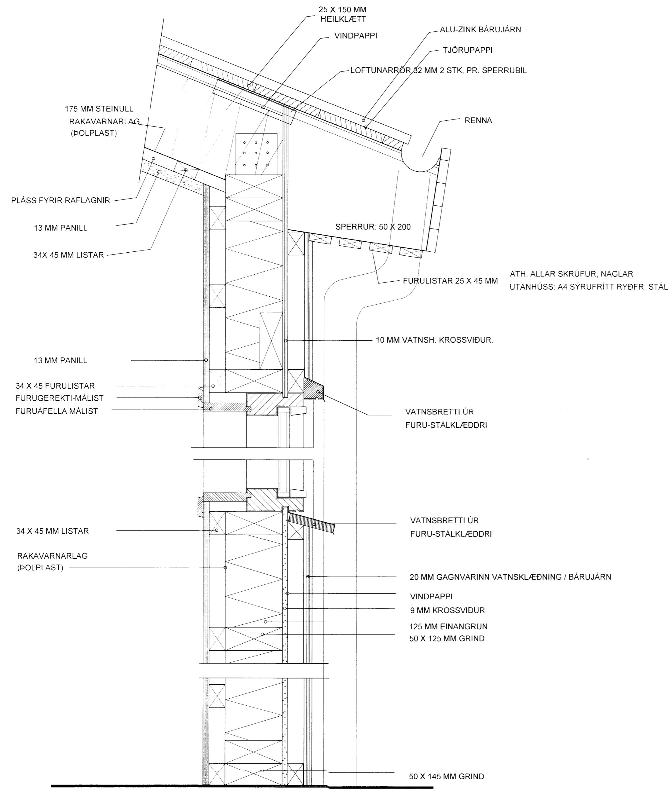
LÓÐRÉTT SNIÐ Í ÚTVEGG OG ÞAK
