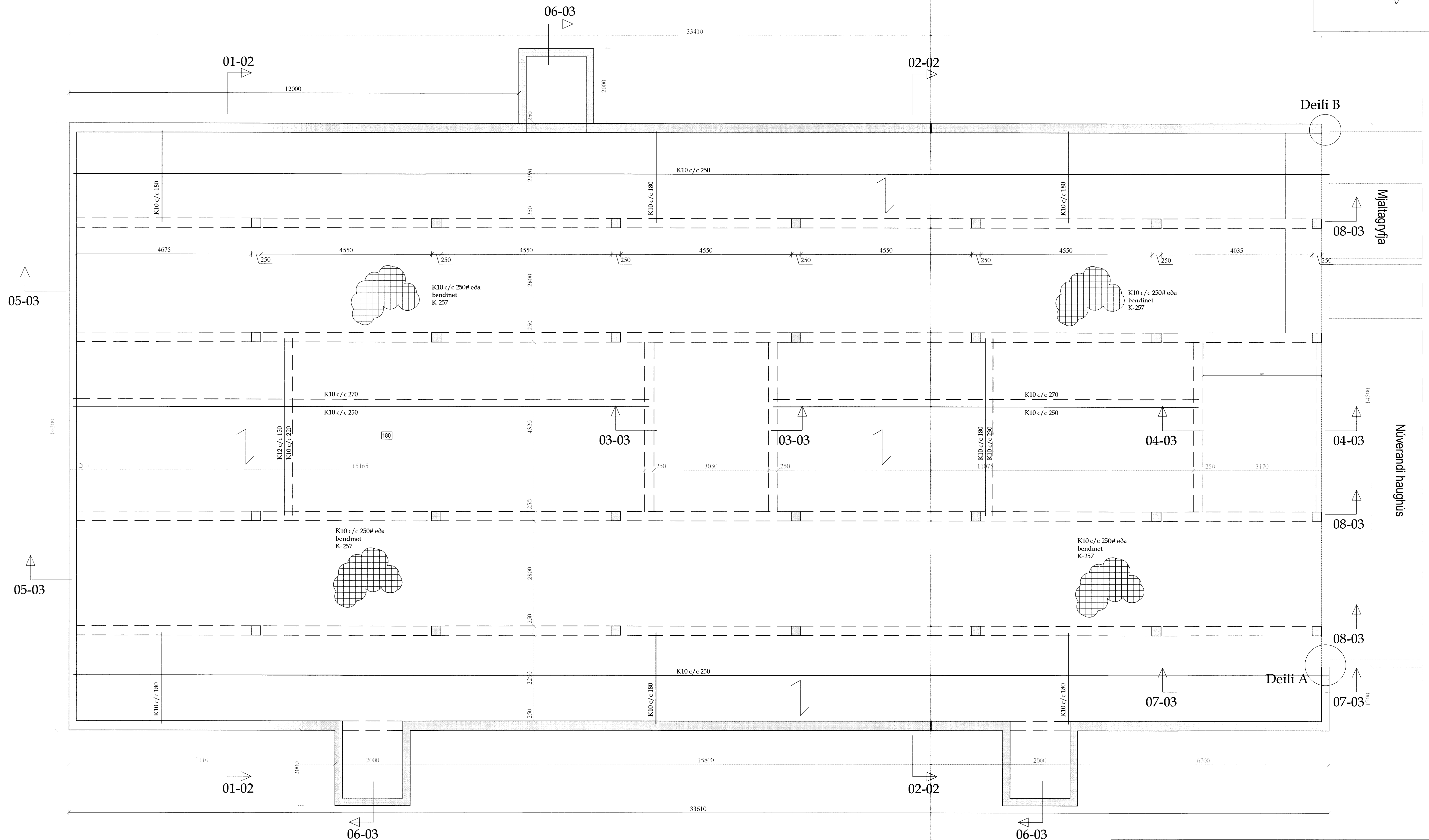
Grunnmynd kjallara mk. 1:50
