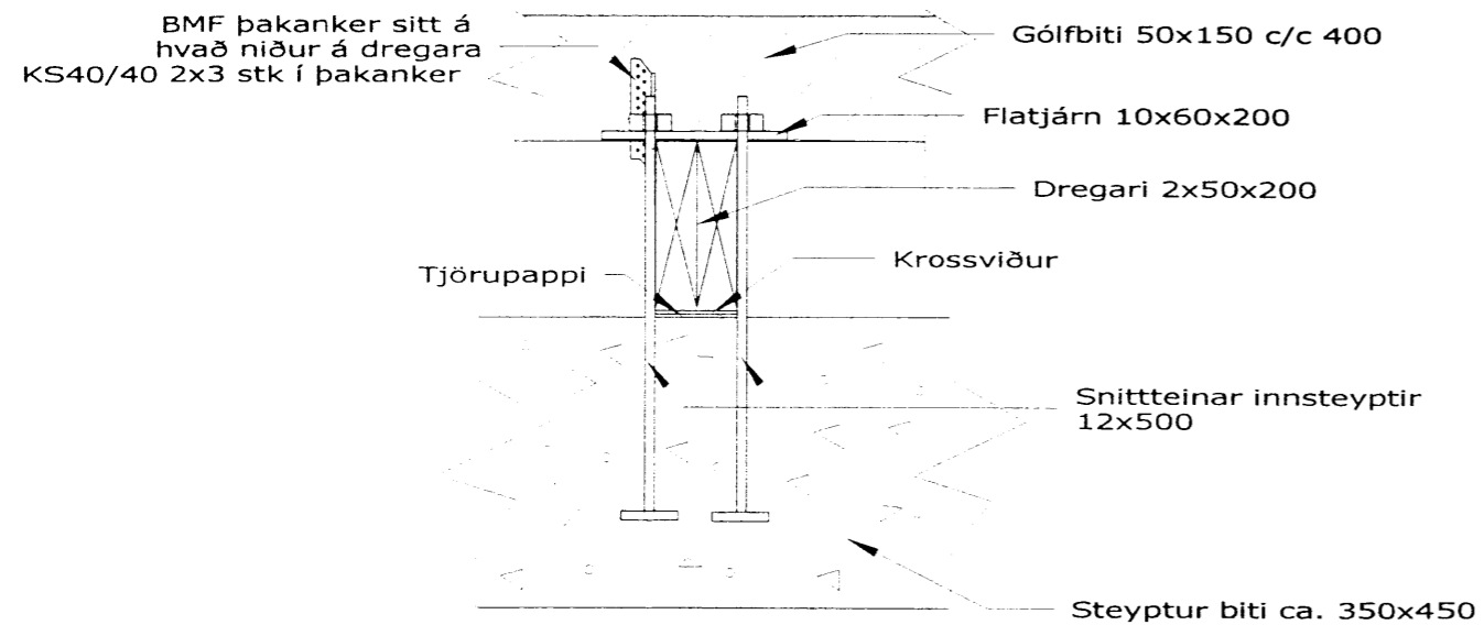
Snið B-B 1:10
