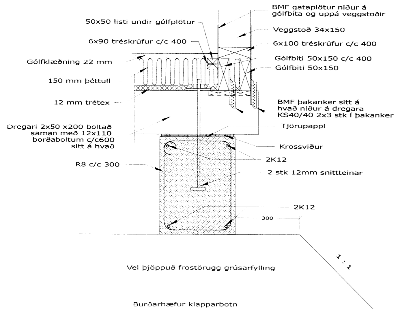
Snið A-A 1:10
