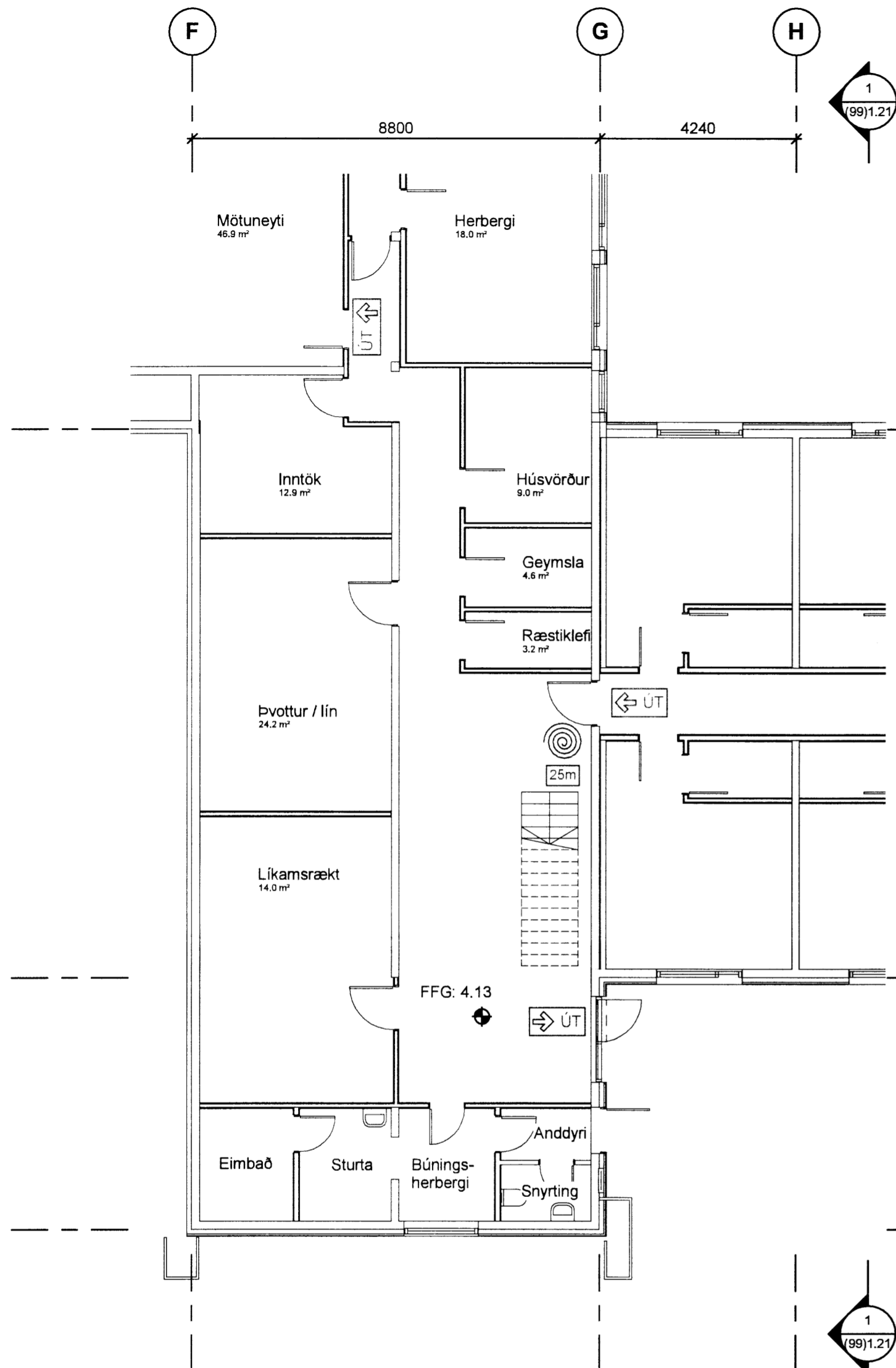
1 Grunnmynd júniorsvíta 1.hæð - núverandi 1 : 100
