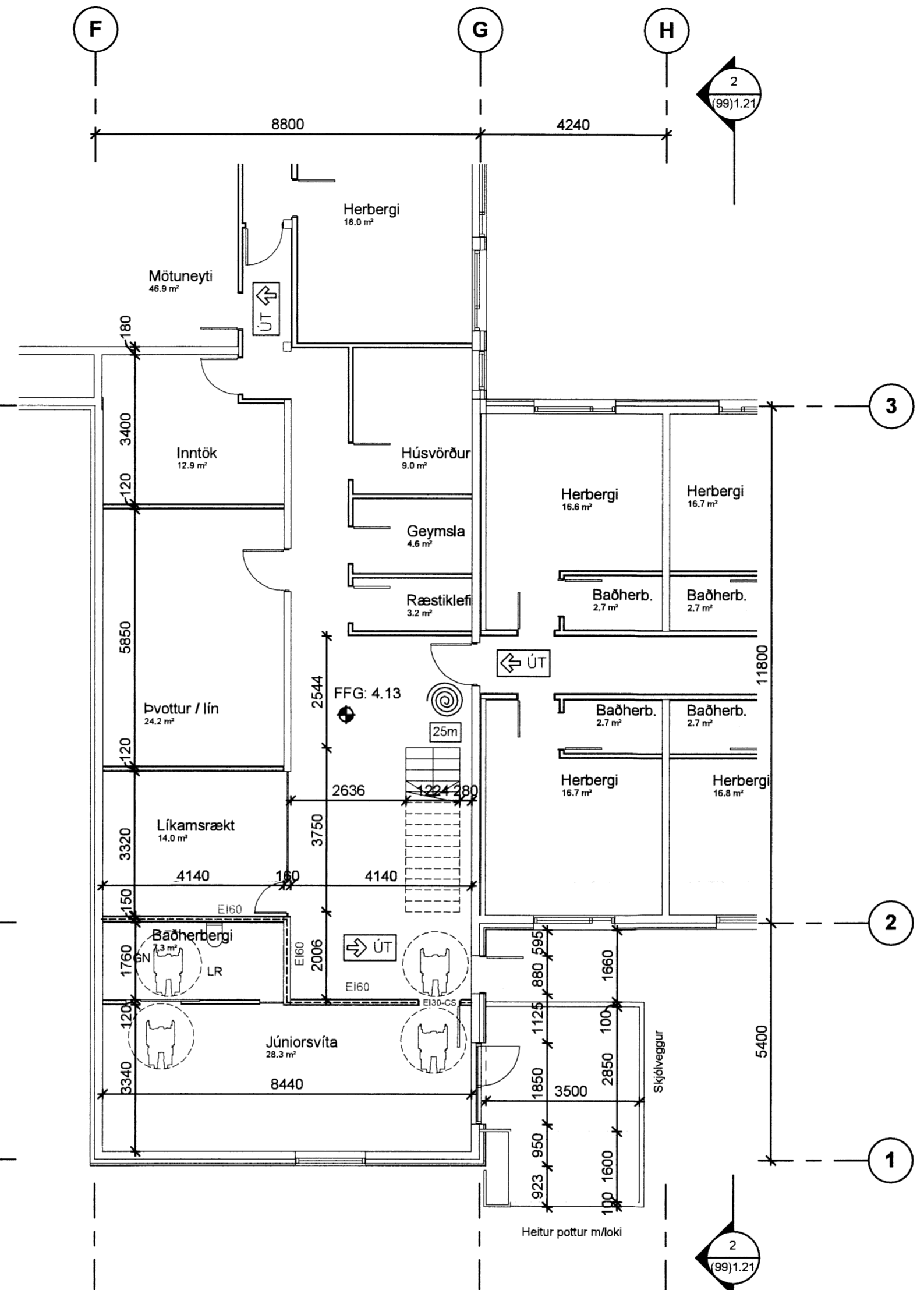
2 Grunnmynd júniorsvíta 1.hæð - breyting 1 : 100
