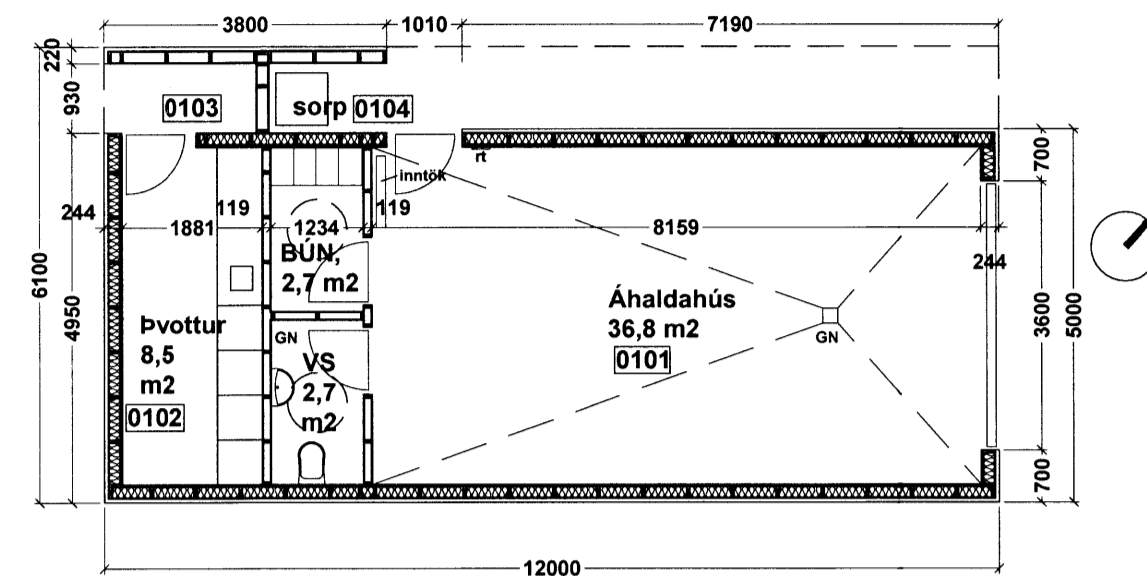
Grunnmynd mkv 1:100
