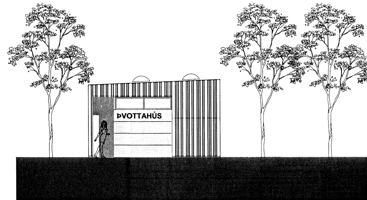
Útlit suðvestur mkv 1:100
