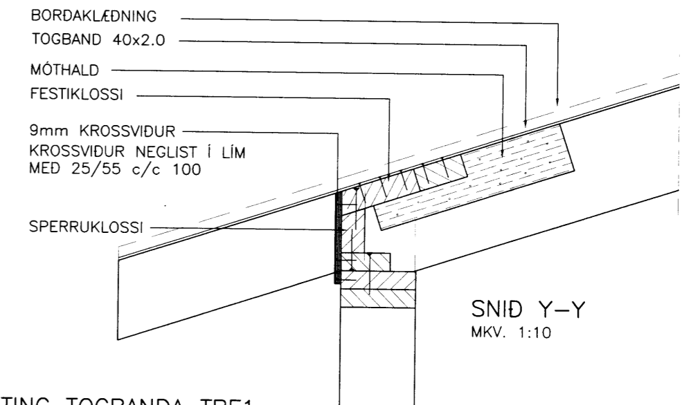
FESTING TOGBANDA TBF1 MKV. 1:20
