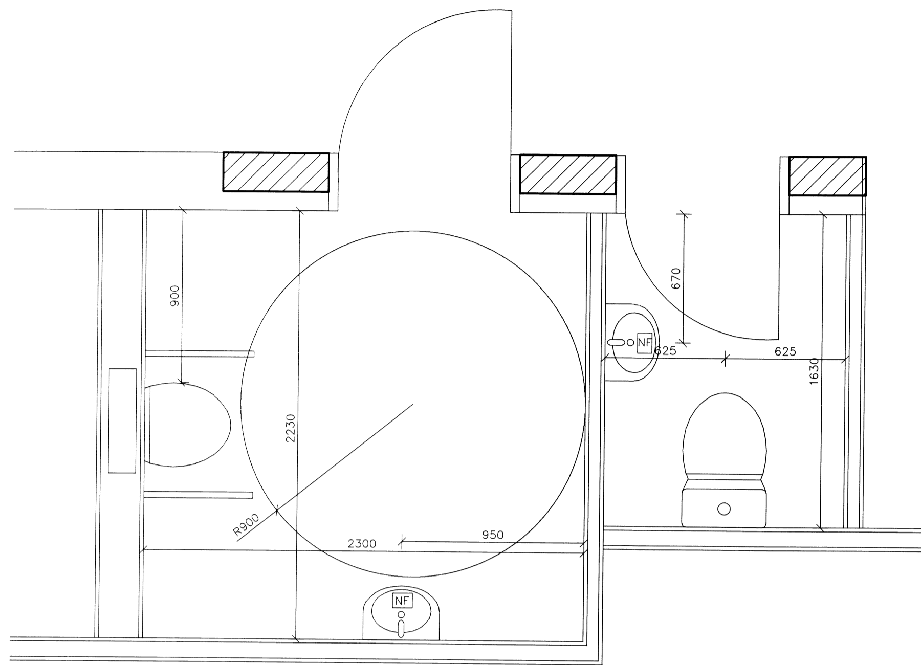
SALERNI - GRUNNMYND MKV. 1:20
