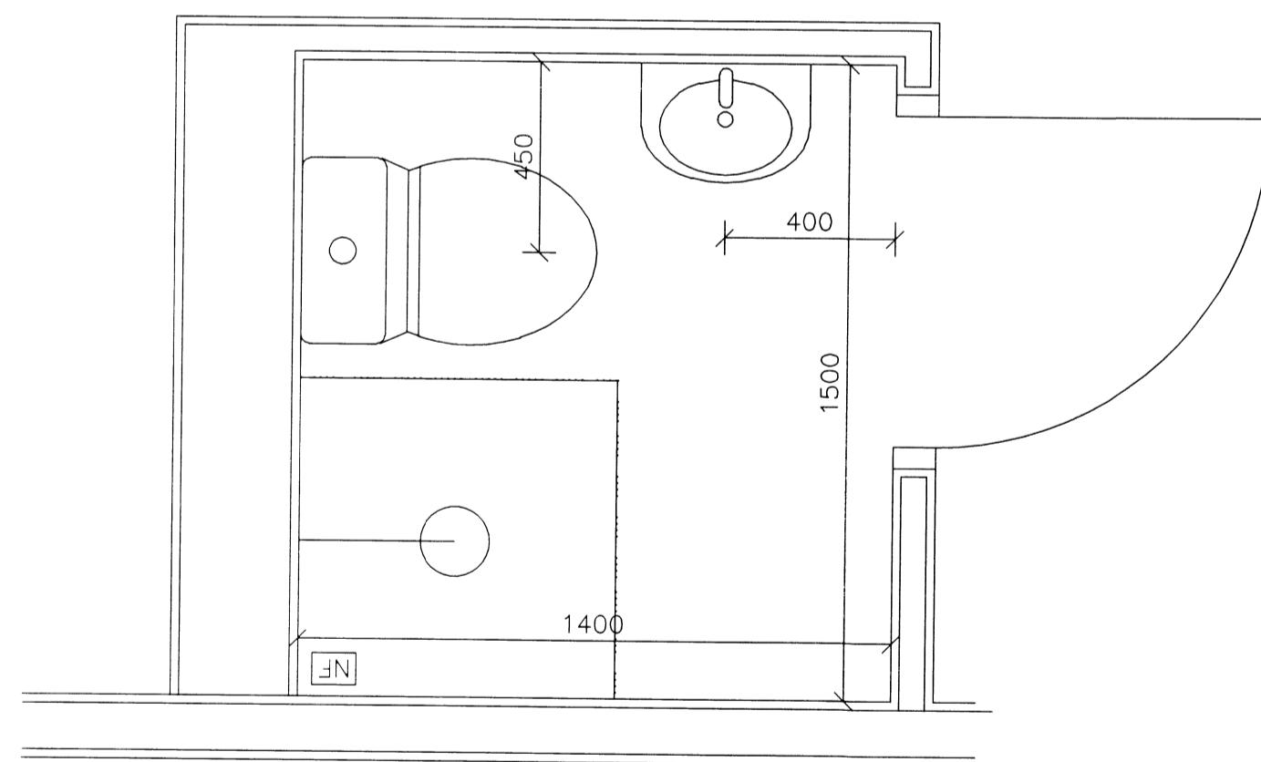
SALERNI Á HERBERGI - GRUNNMYND MKV. 1:20
