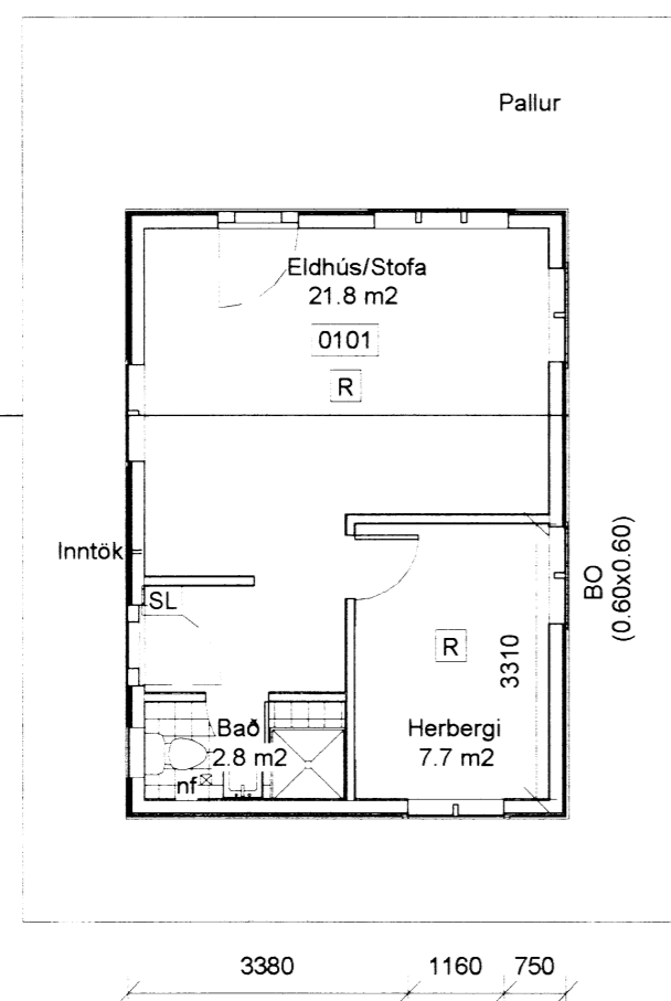
Grunnmynd M: 1:100
