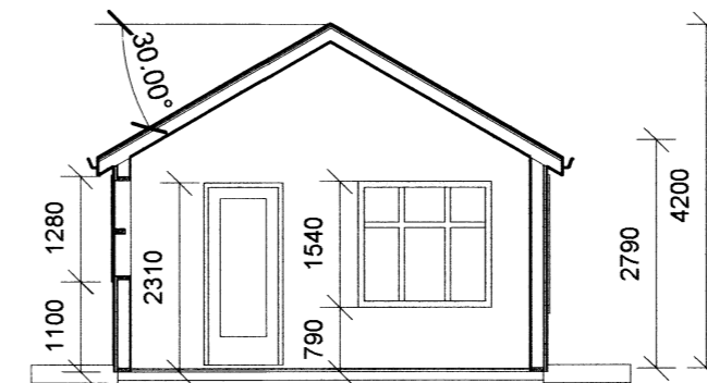
Snið A-A M: 1:100
