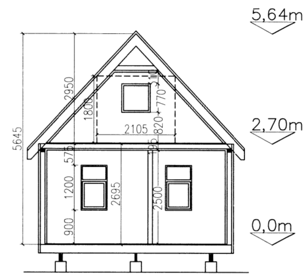
Snið A
