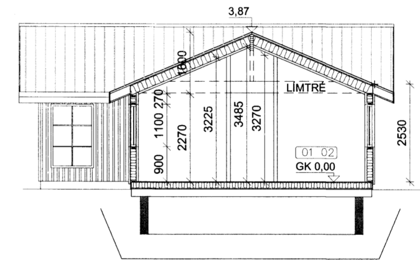
SNID B-B 1:100
