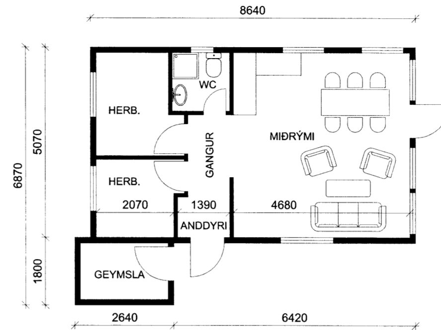
NÚVERANDI GRUNNMYND 1:100
