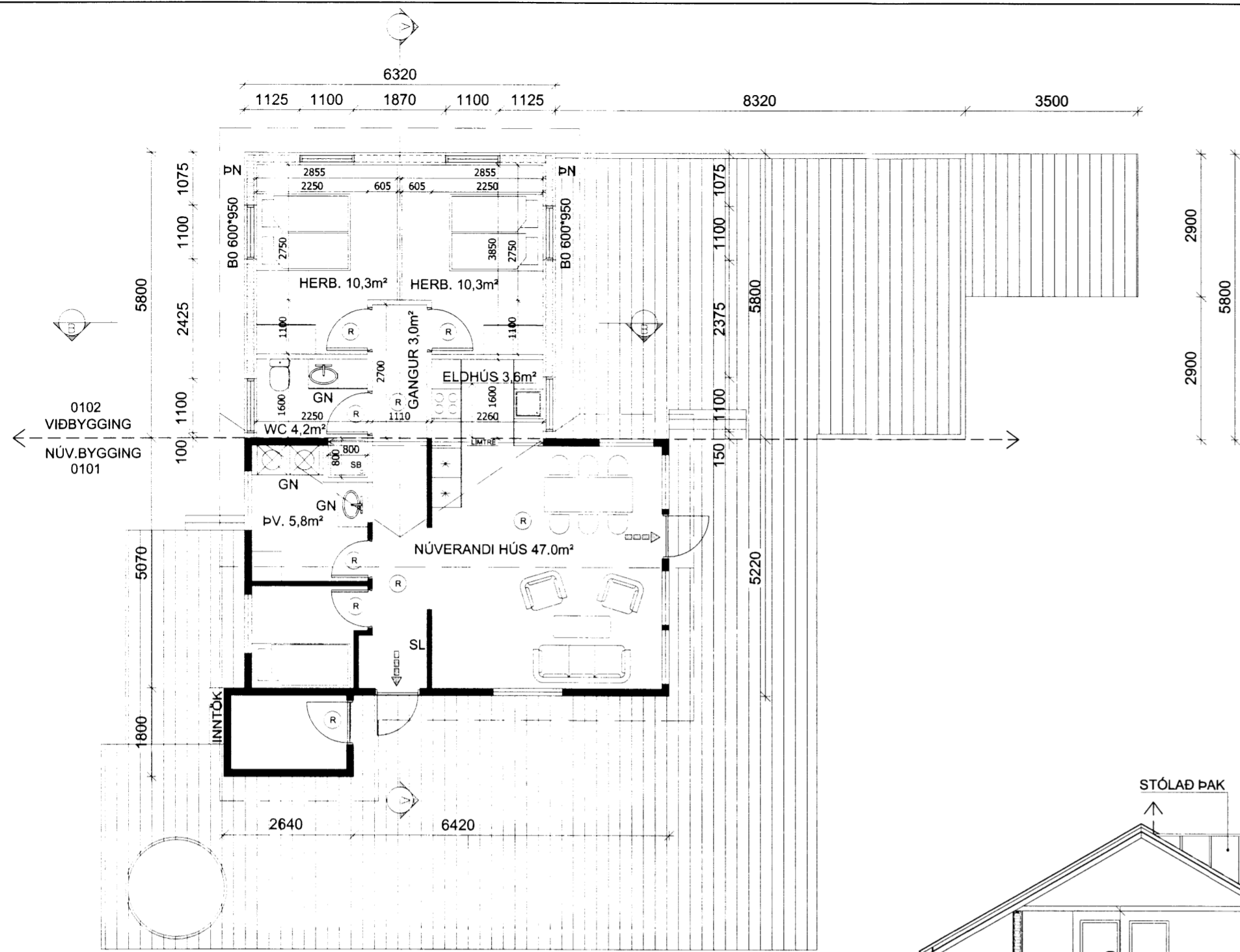
GRUNNMYND 1:100 86.2m²
