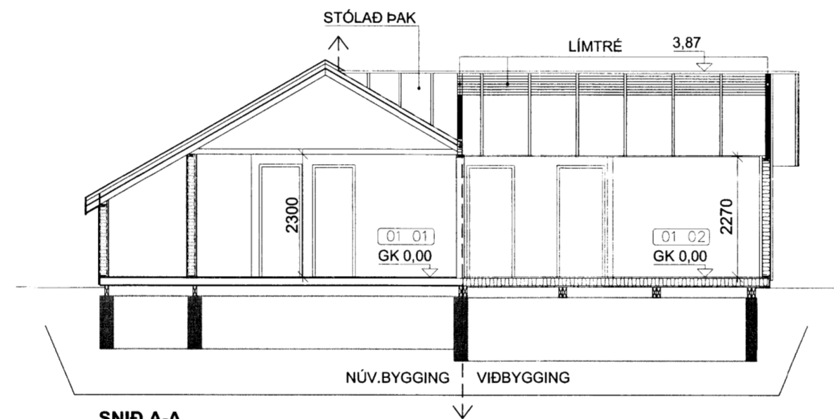
SNID A-A 1:100
