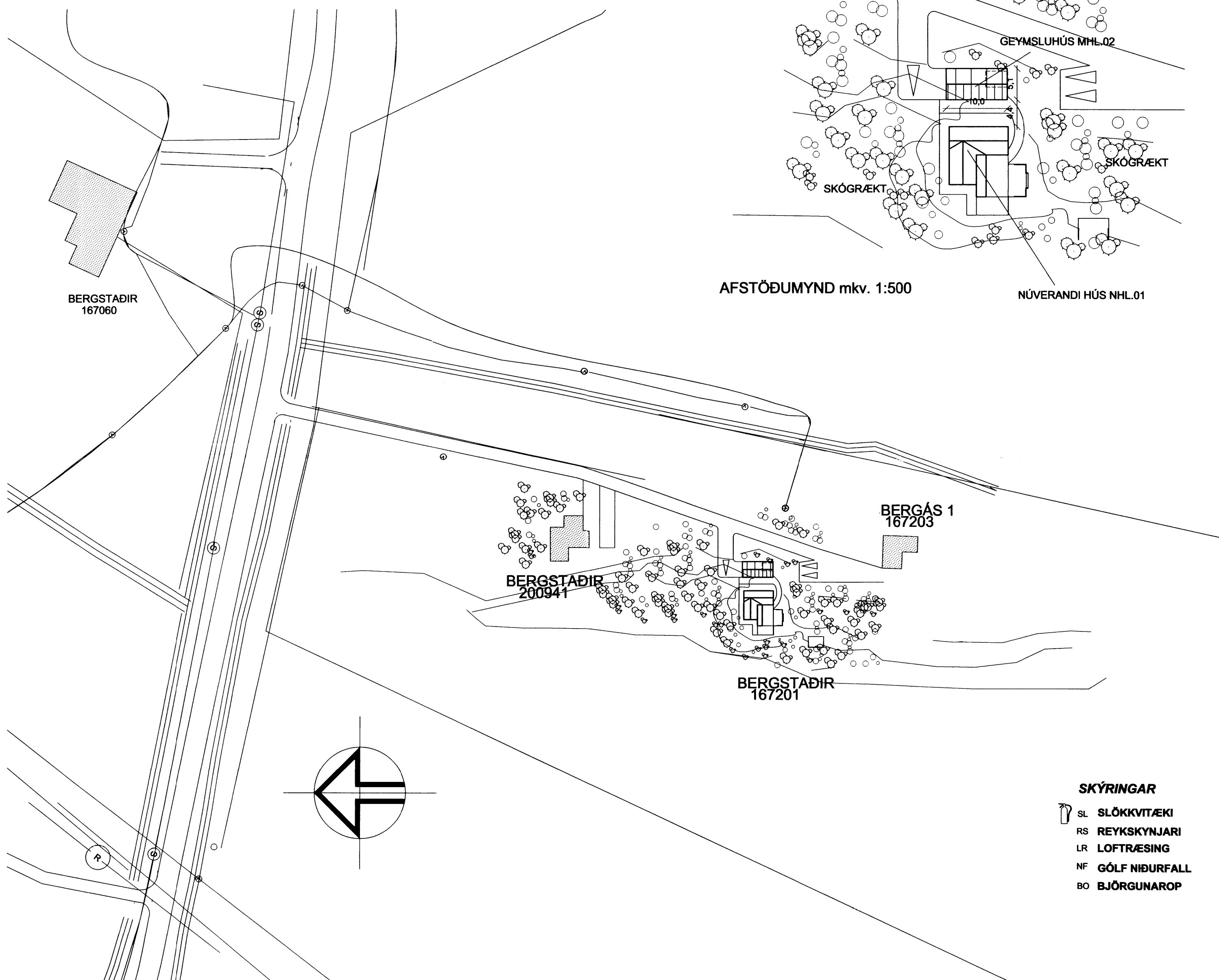
AFSTÖÐUMYND mkv. 1:1000
