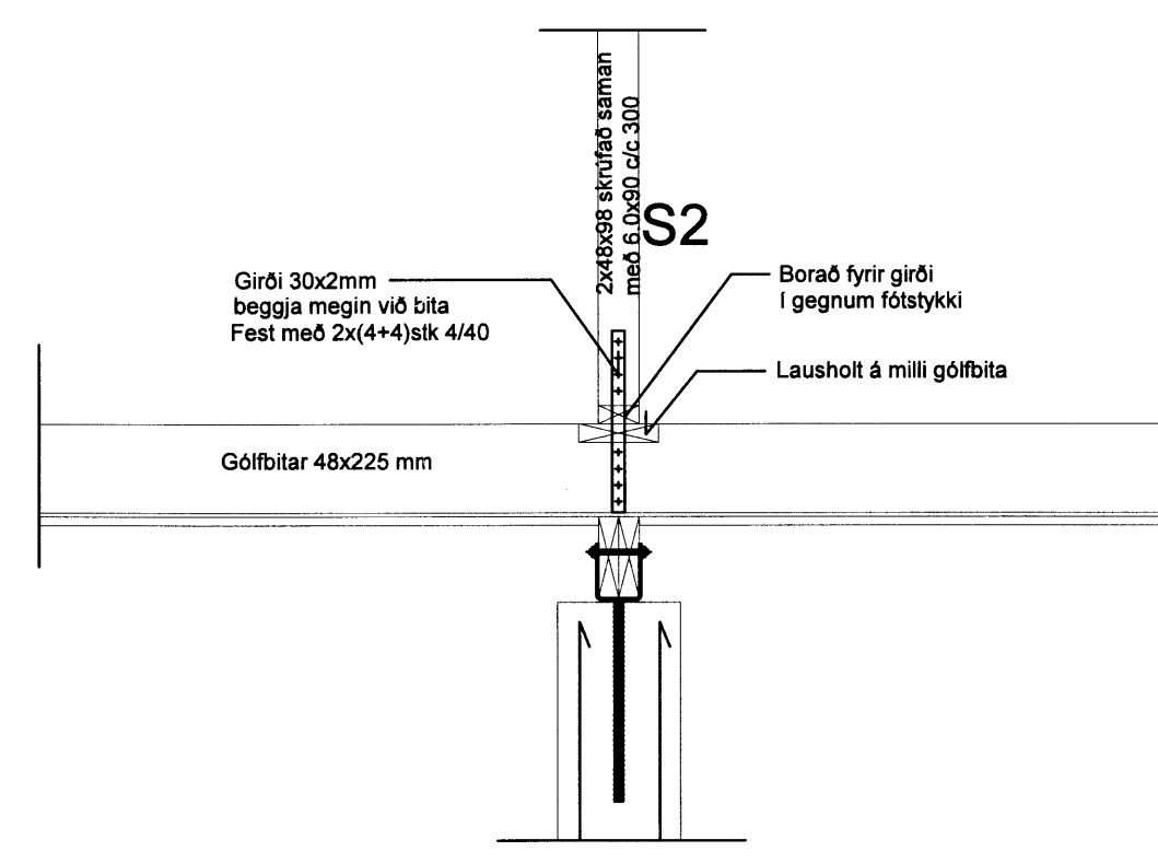
Snið G
