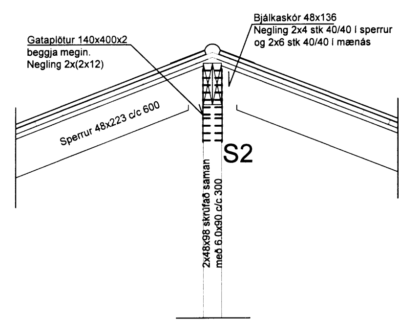
Snið E
