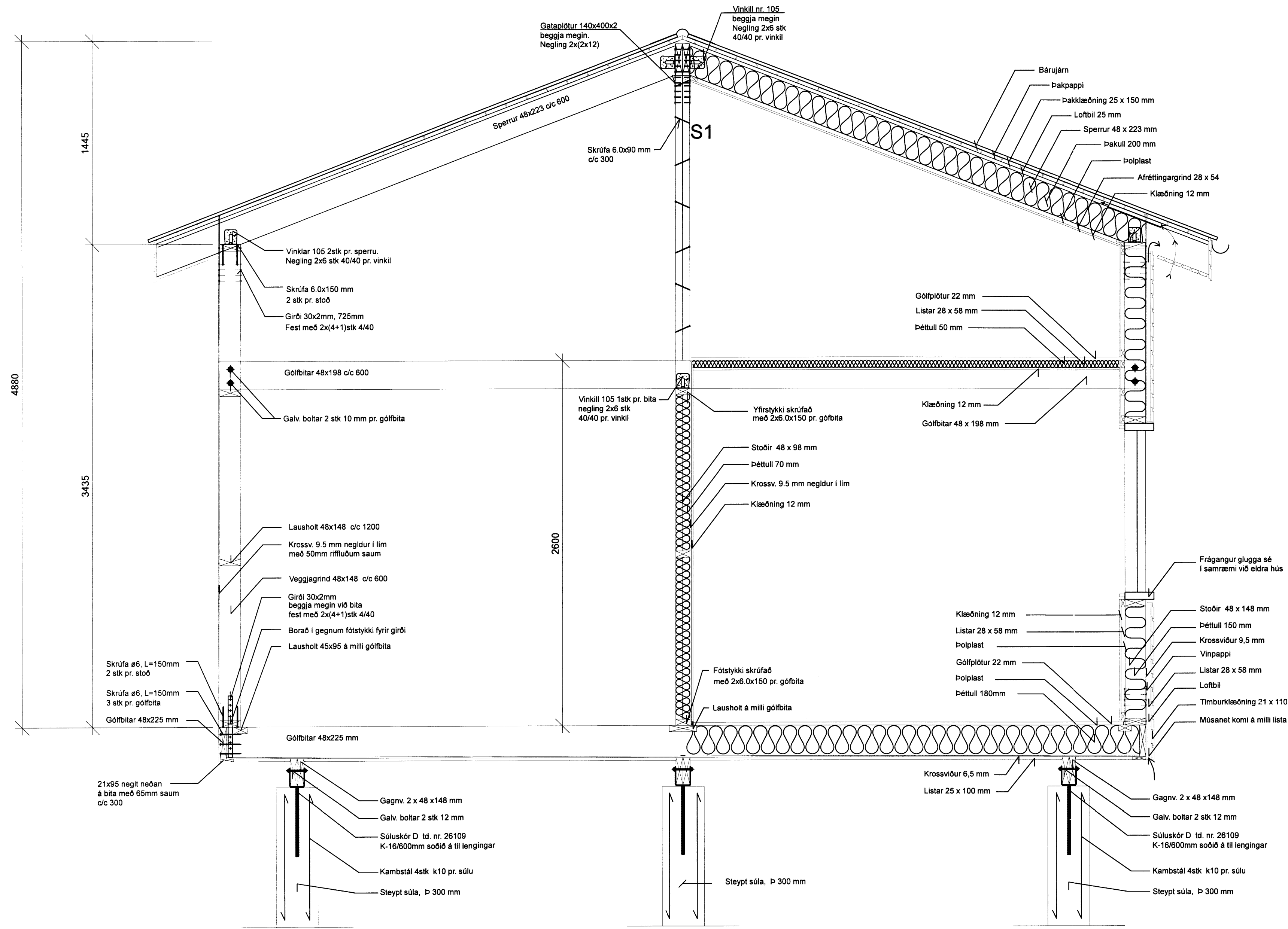
Snið D-D
