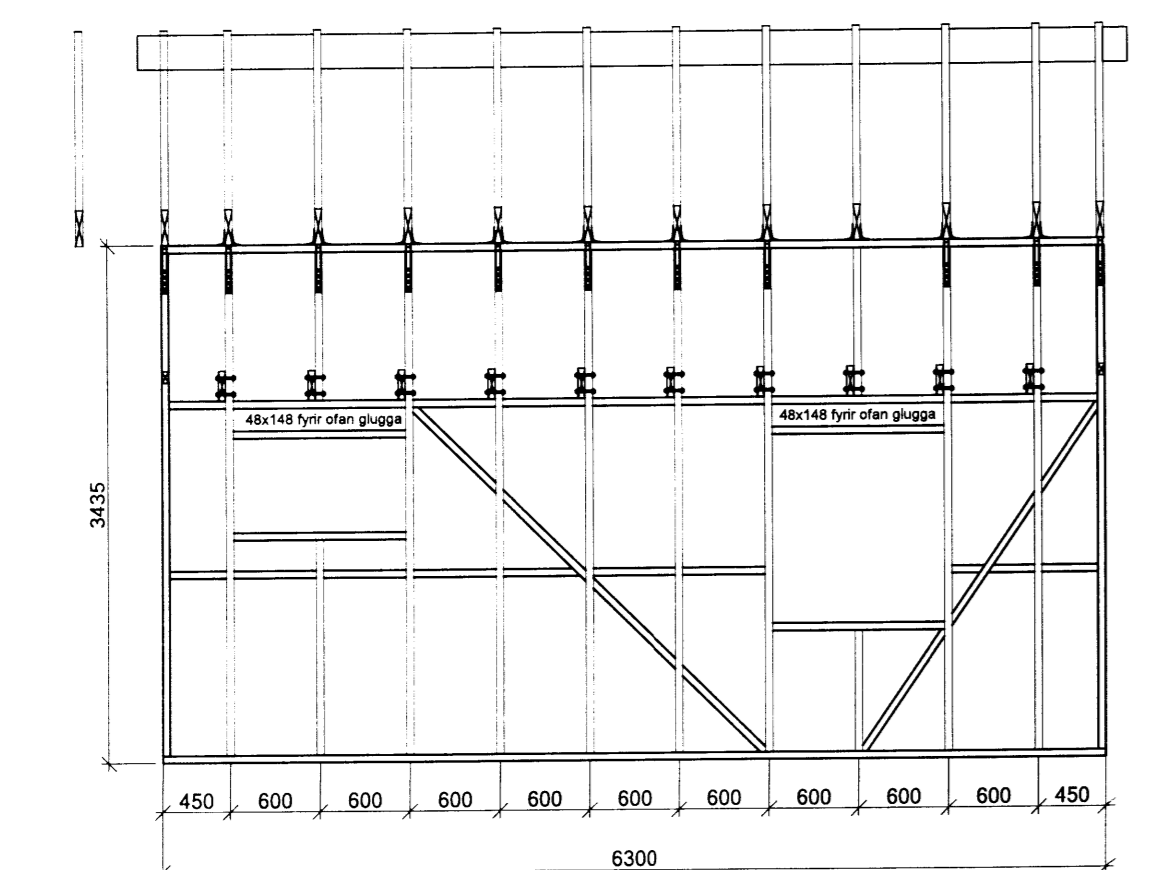
Veggjagrind austur
