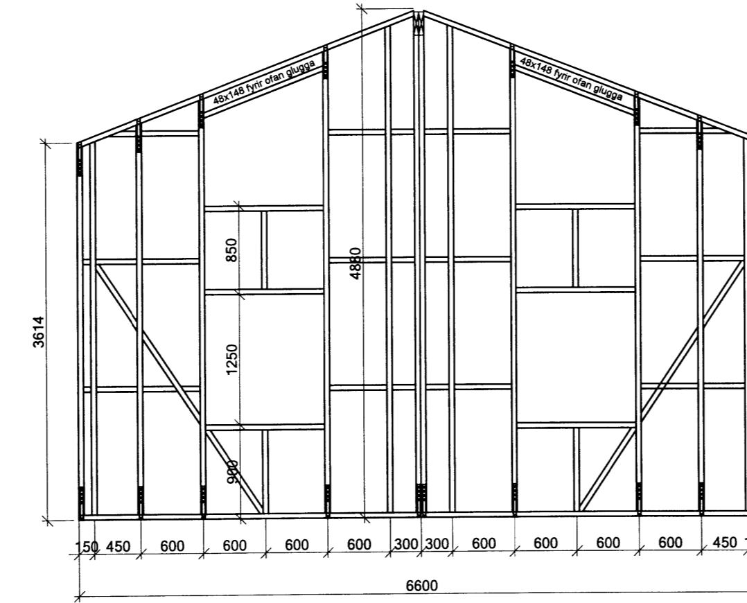
Veggjagrind norður
