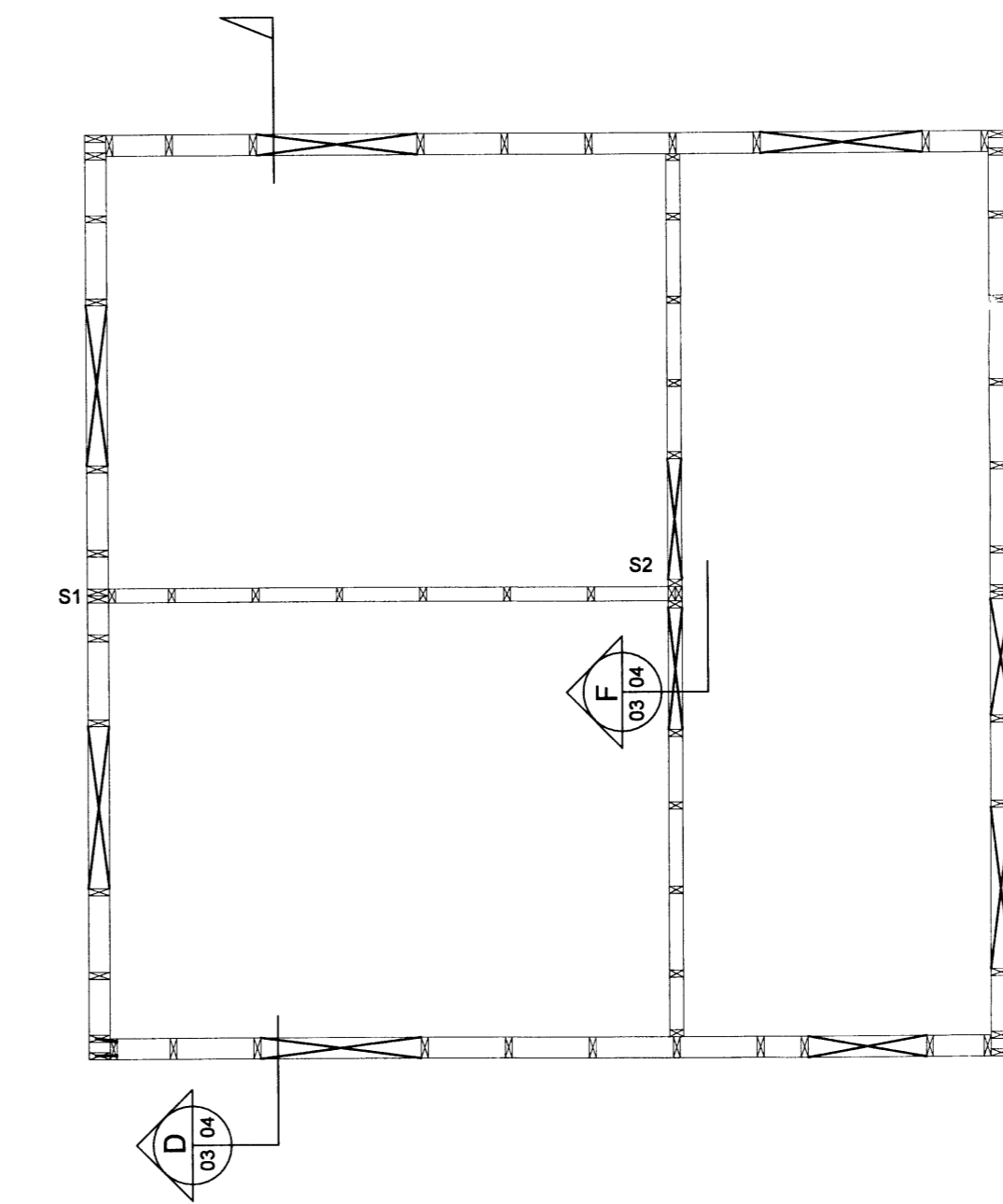
Veggjagrind grunnmynd
