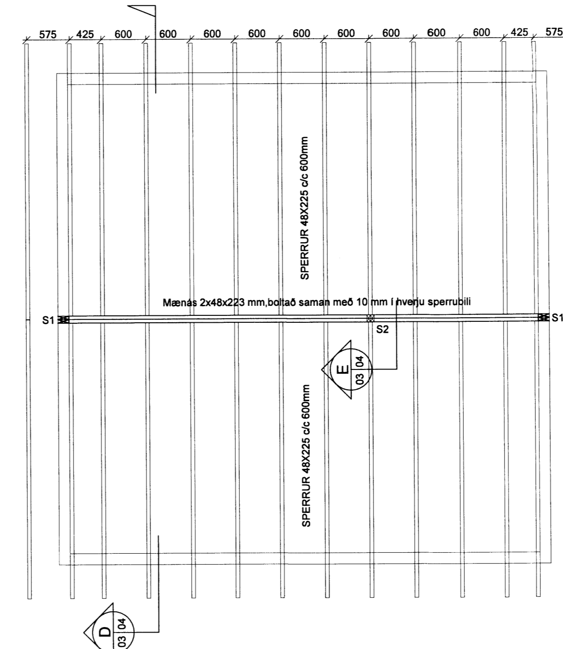
Sperrur
