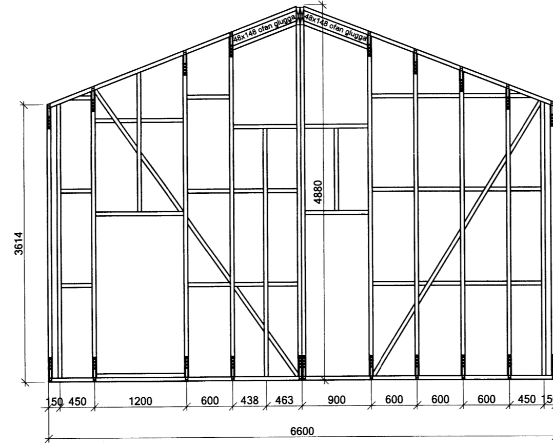
Veggjagrind suður
