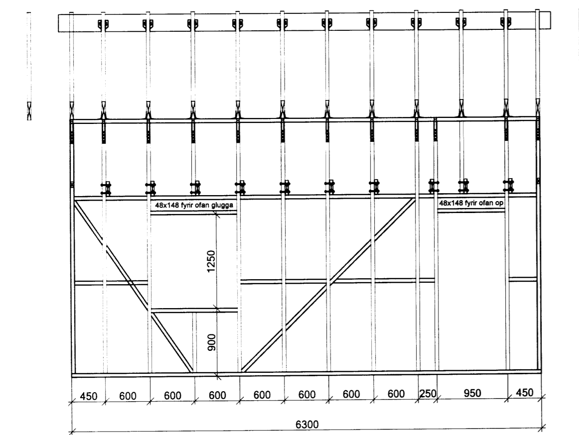
Veggjagrind vestur
