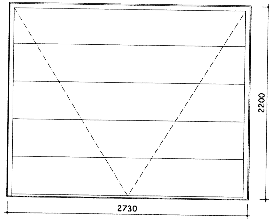
G13 1 stk. bílskúrshurð, flekar Slick (slétt skv. bæklingi) RAL 7016
