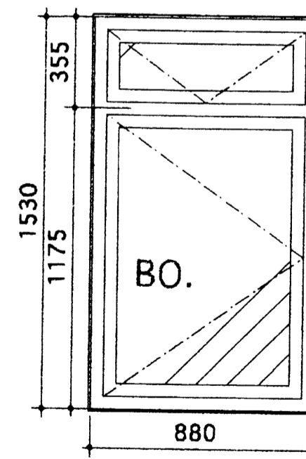
G8 3 stk. Opnanlegt fag. Björgunarop 1100 x 780 mm
