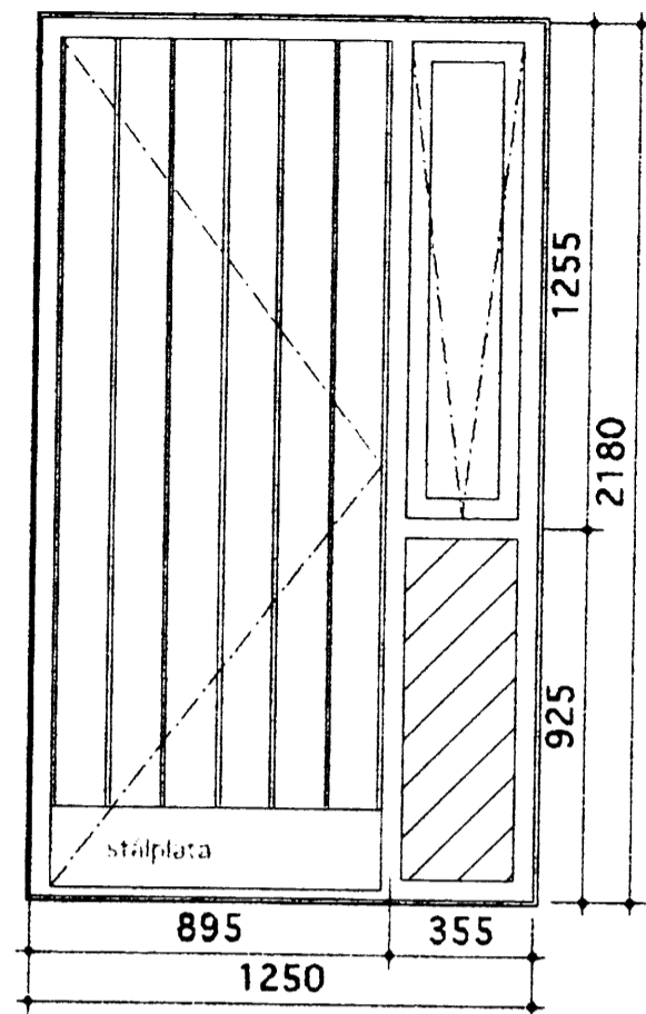
G10 1 stk. hurð opnasti út. Rásaður viður (lóðrétt) í hurðarspjaldi cc ca 120mm. Opnanlegt fag.
