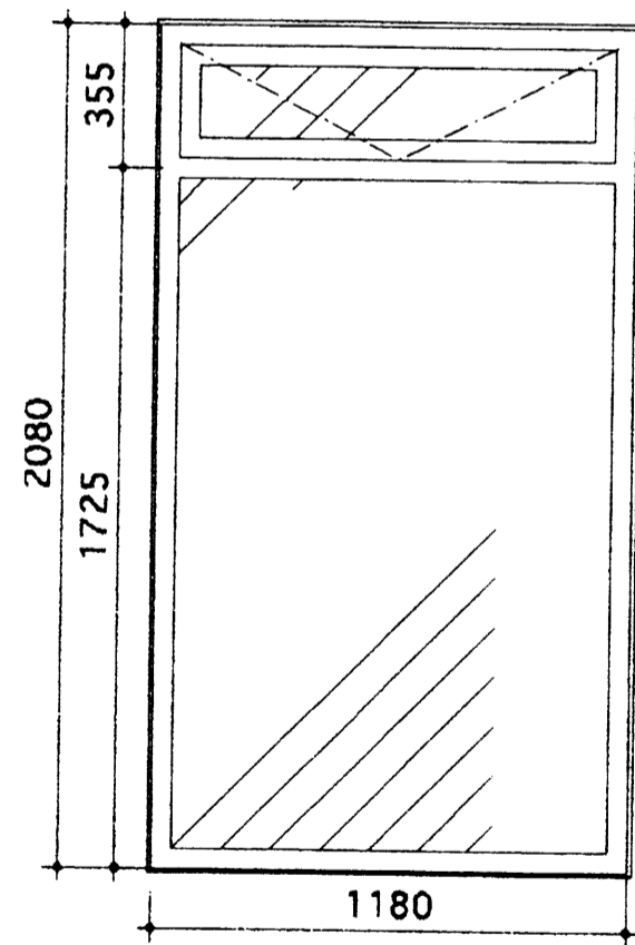
G5 1 stk. Opnanlegt fag.
