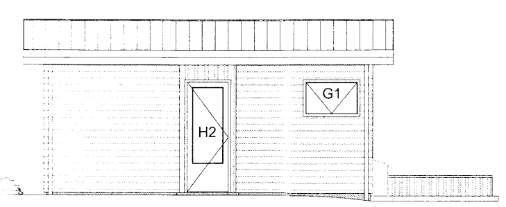
ÚTLIT NORD-VESTUR 1:100
