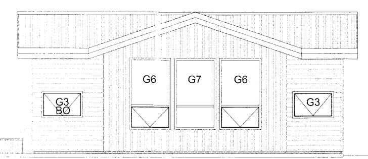
ÚTLIT SUÐ-AUSTUR 1:100
