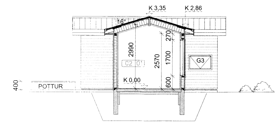
SNÍÐ D-D 1:100
