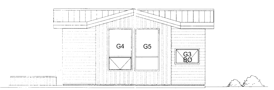
ÚTLIT SUÐ-AUSTUR 1:100
