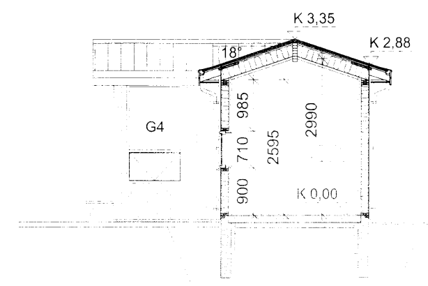
SNÍÐ C-C 1:100
