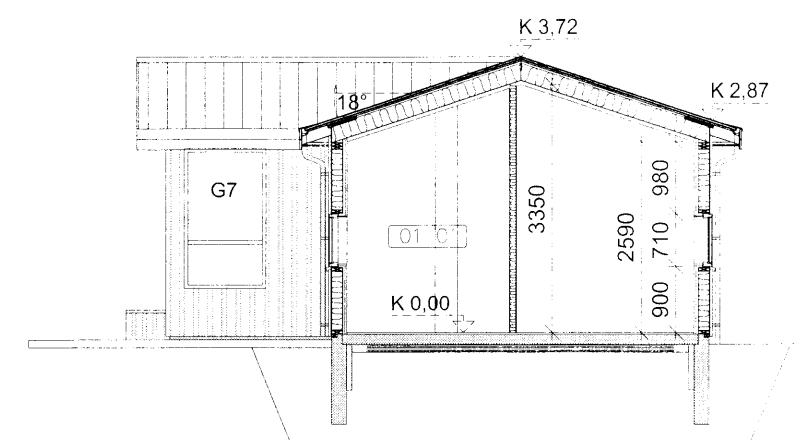
SNÍÐ A-A 1:100
