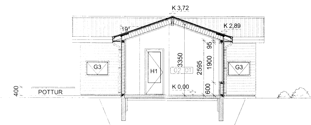
SNÍÐ B-B 1:100
