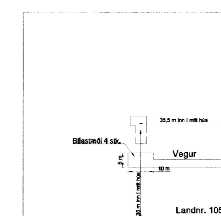
AFSTÖÐUMYND MKV. 1:1000
