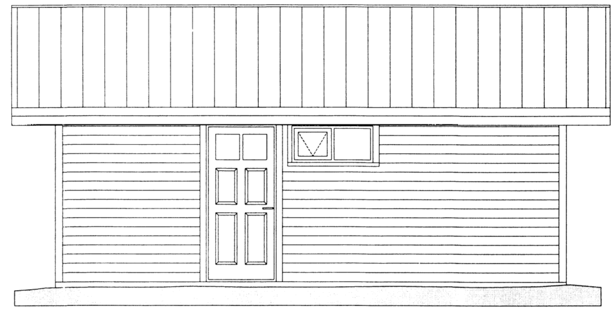
AUSTURHLIÐ Mkv. 1:50
