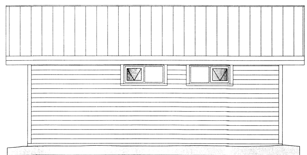
VESTURHLIÐ Mkv. 1:50
