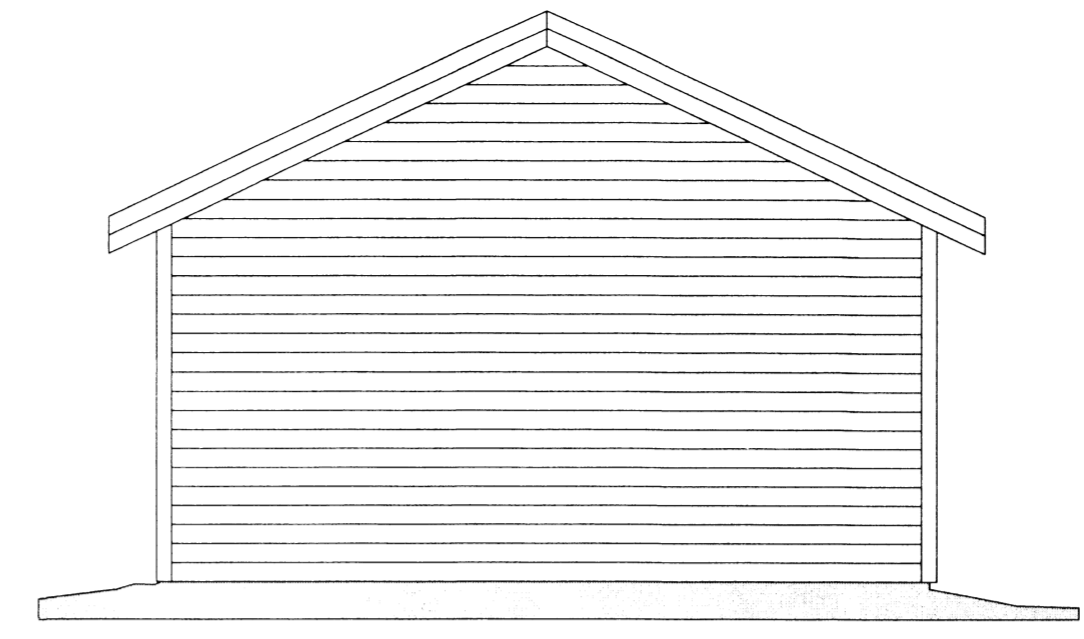
SUÐRUGAFL Mkv. 1:50
