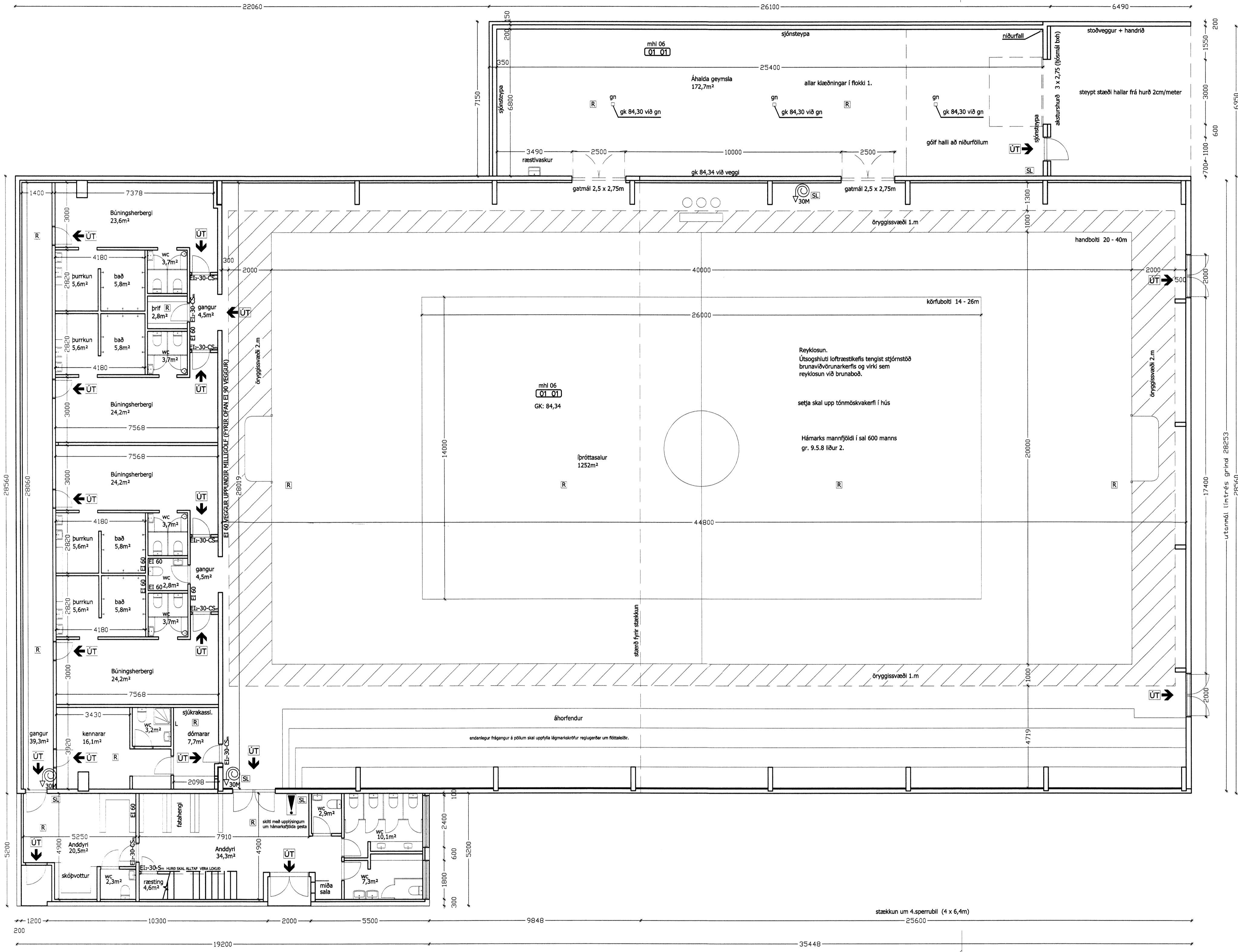
GRUNNMYND 1. HÆÐ 1:100
