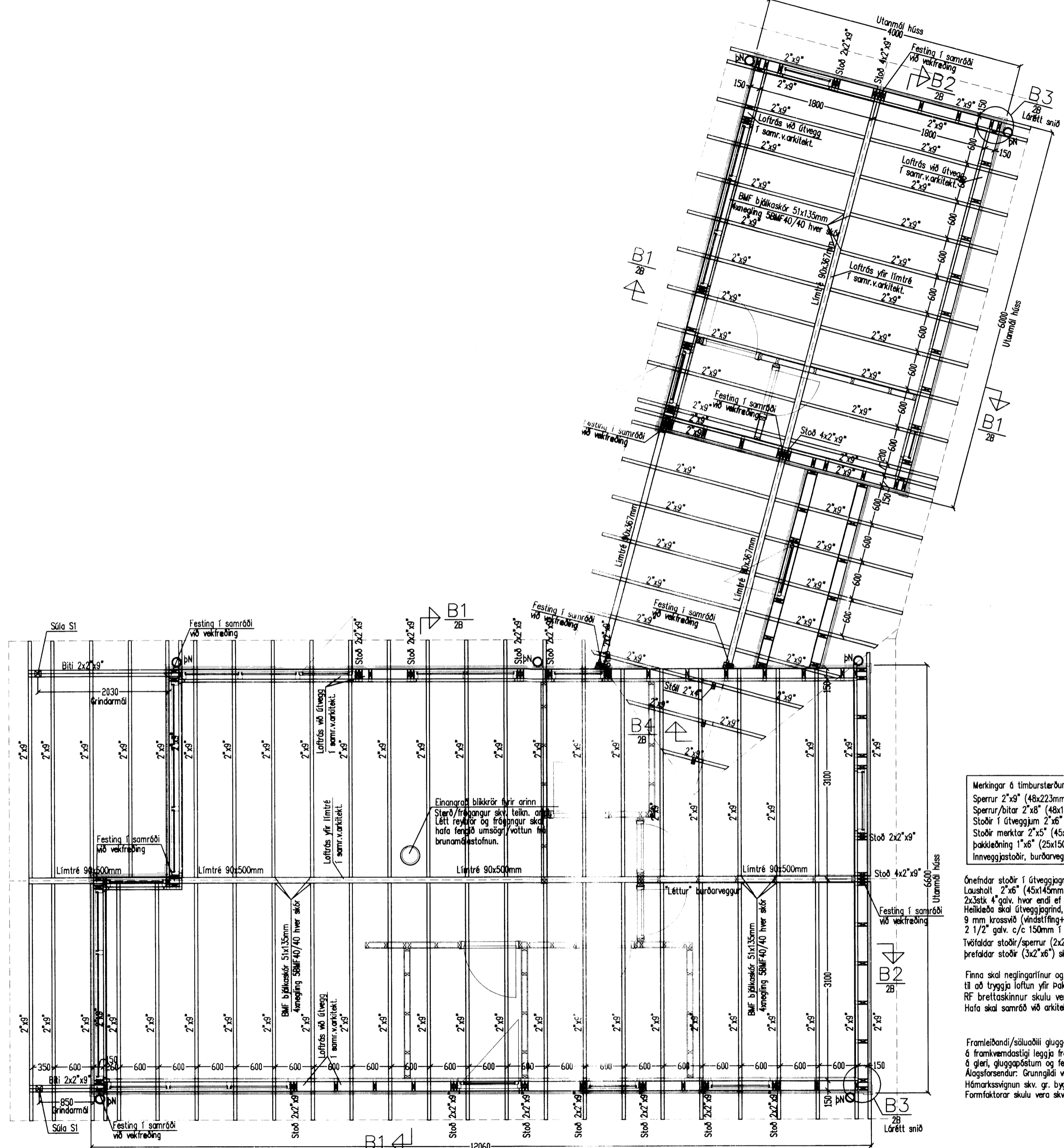
Grunnmynd Þakvirkis 1:50
