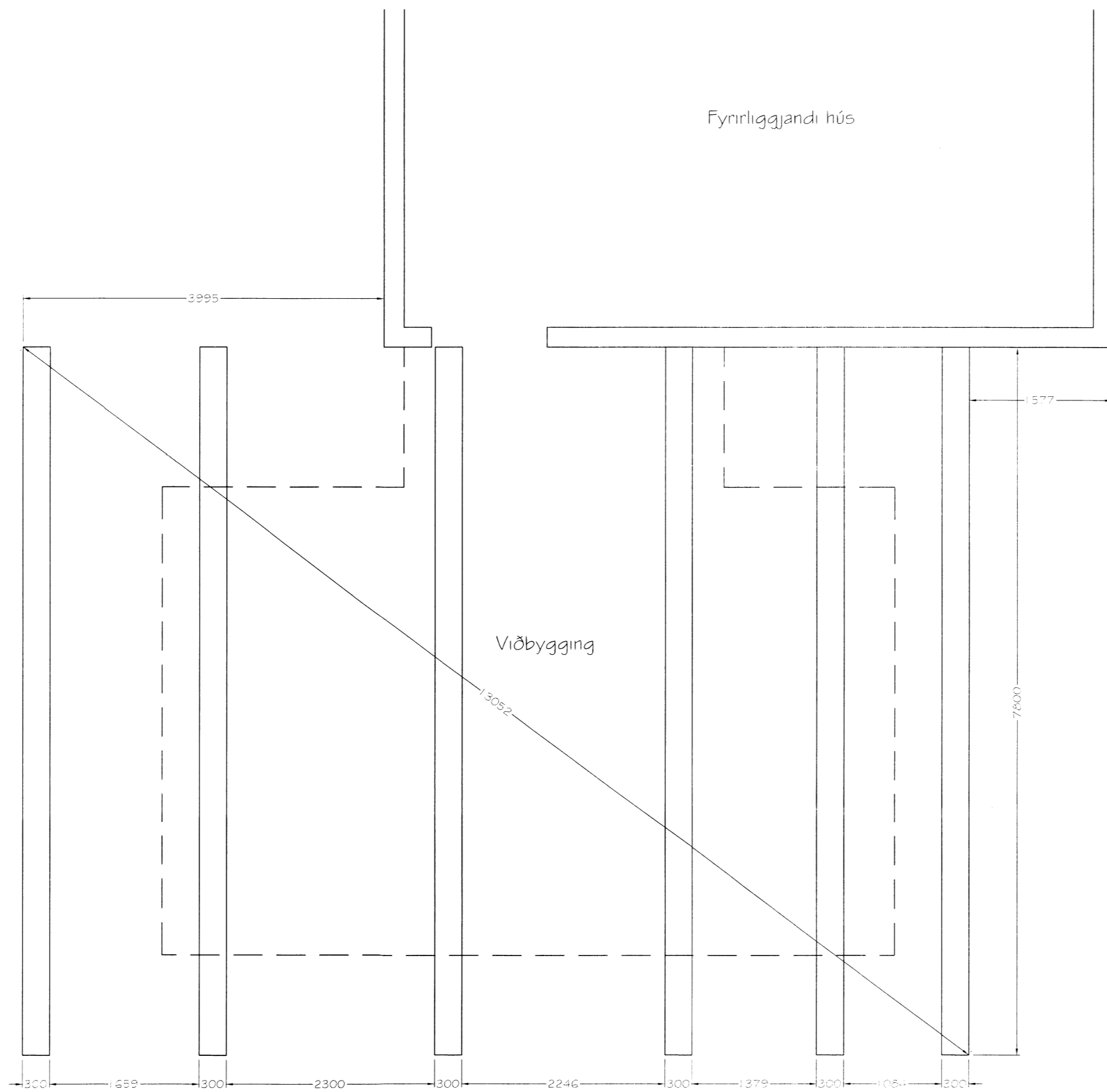
Grunnmynd undirstöður
