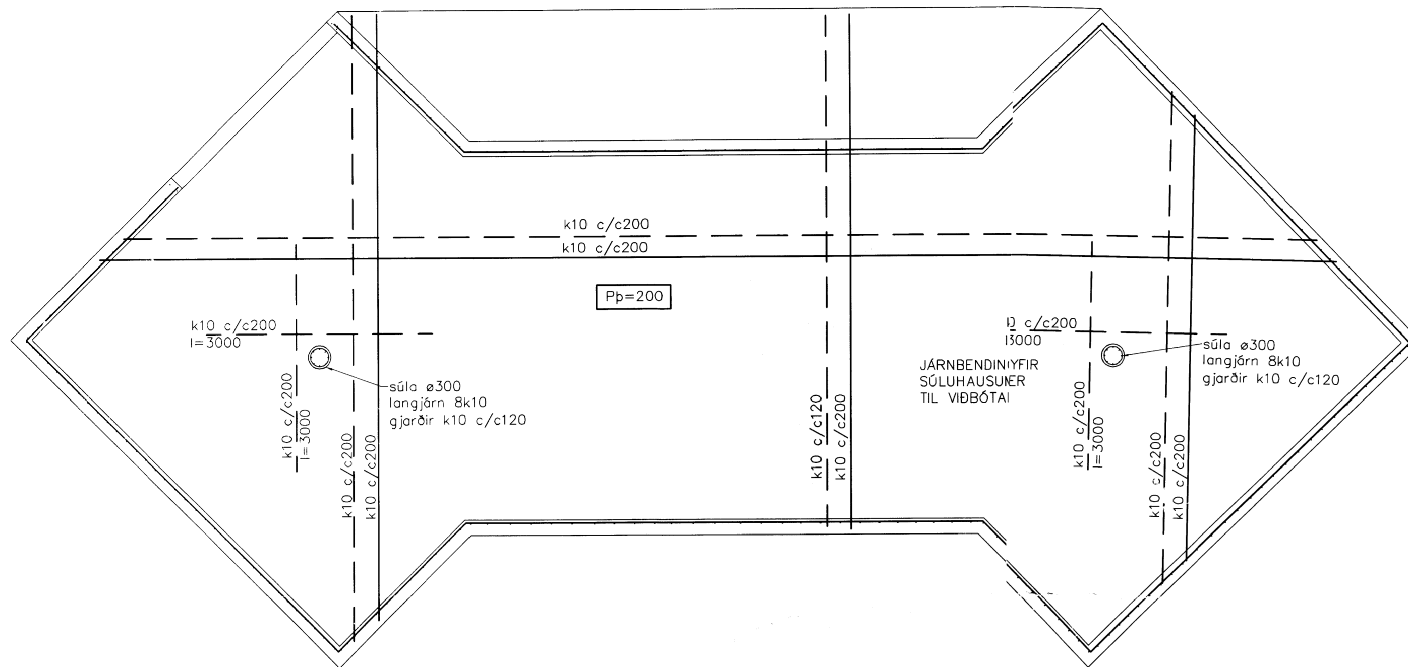
GRUNNMYND 1:50
