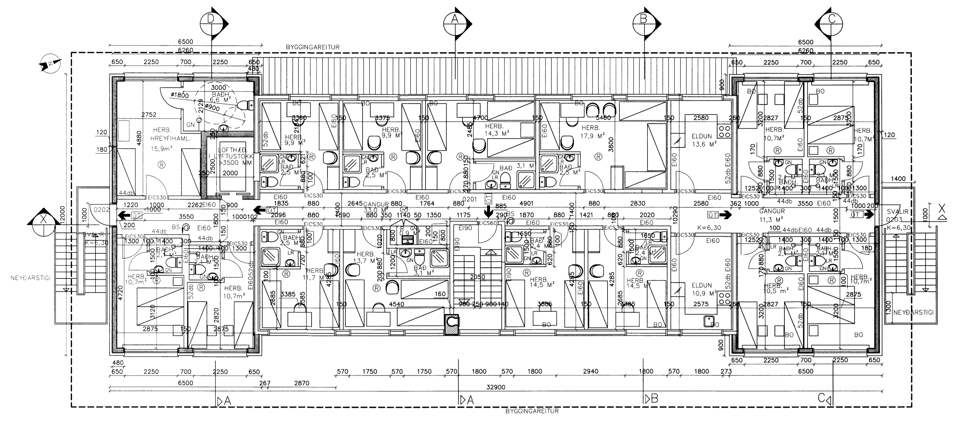
GRUNNMYND 3.HÆÐ MKV.1:100
