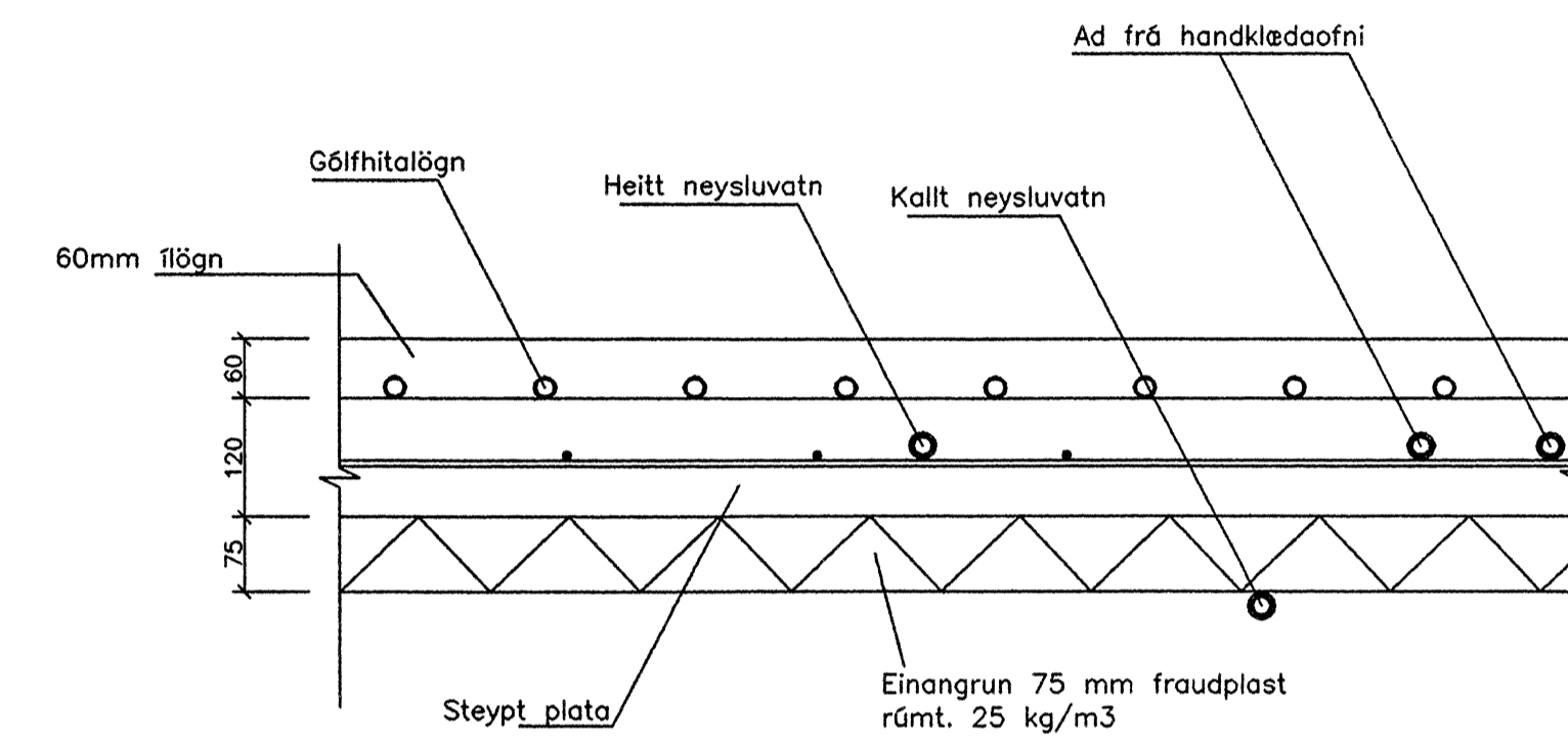
STADSETNING HITA OG VATNSLAGNA Í BOTNPLÖTU ÍBÚÐARHLUTA
