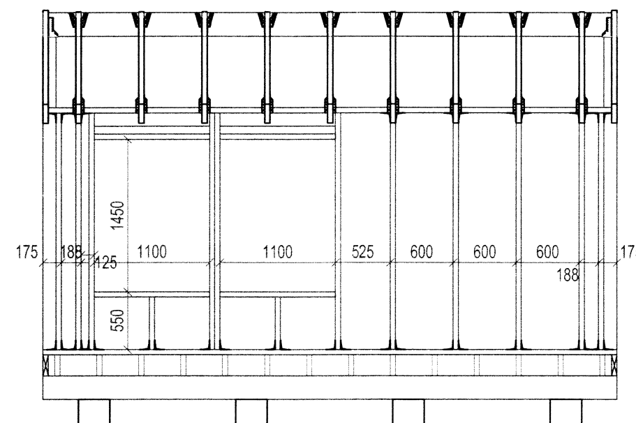
Ásýnd mót suðri mkv. 1:50
