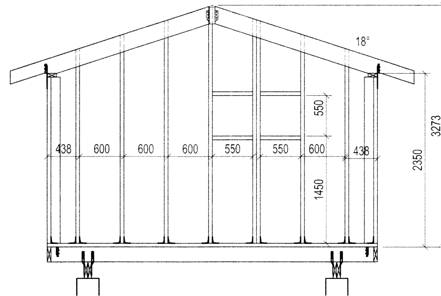
Ásýnd mót austri mkv. 1:50
