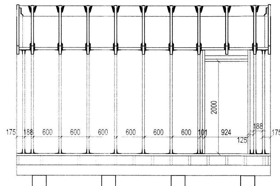
Ásýnd mót norðri mkv. 1:50
