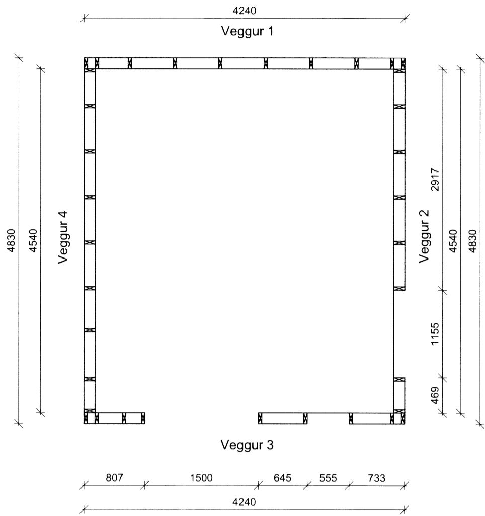
Grunnmynd veggja M 1:50
