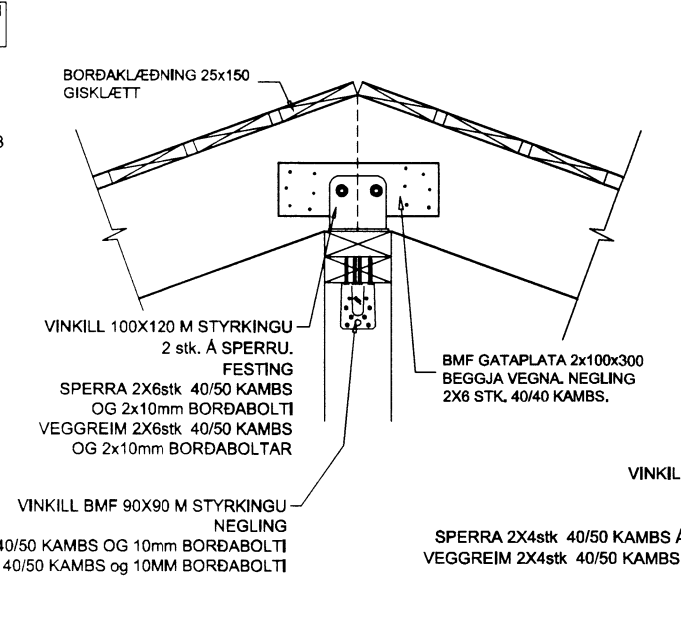
Festing F2 mkv. 1:10
