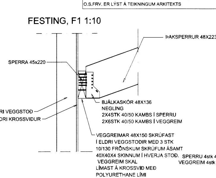
Festing F1 mkv. 1:10
