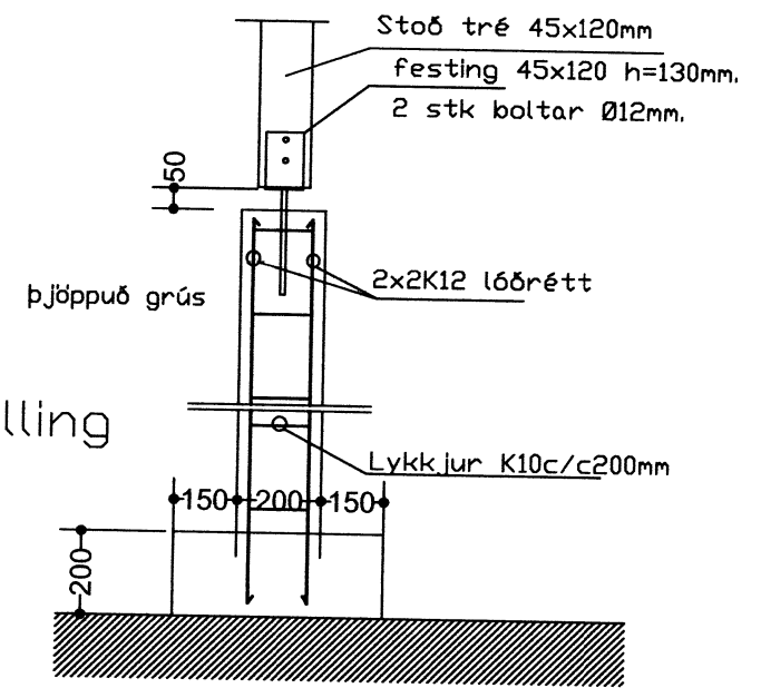
Súla S1 1:20
