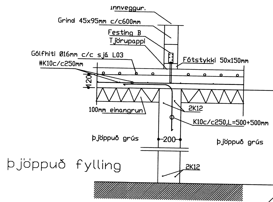
Snið B 1:20
