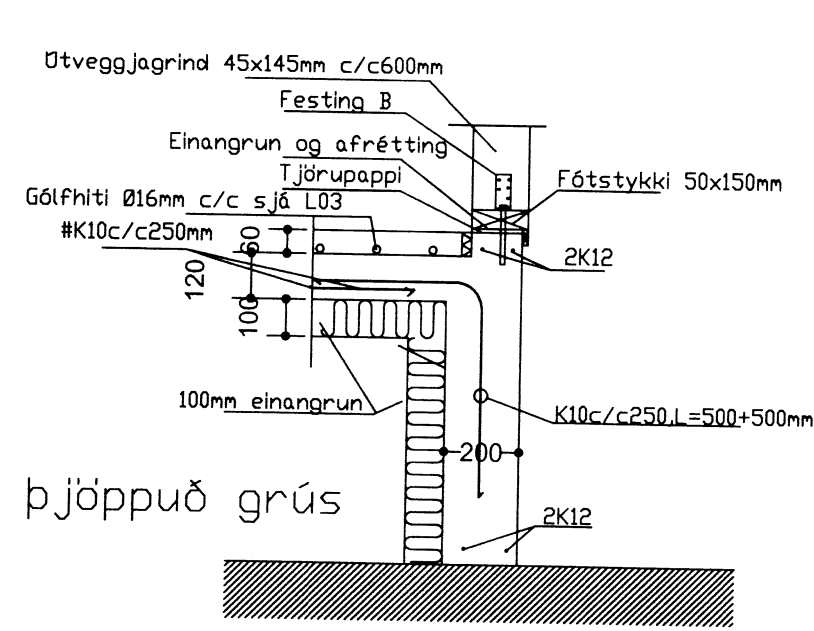
Snið A 1:20
