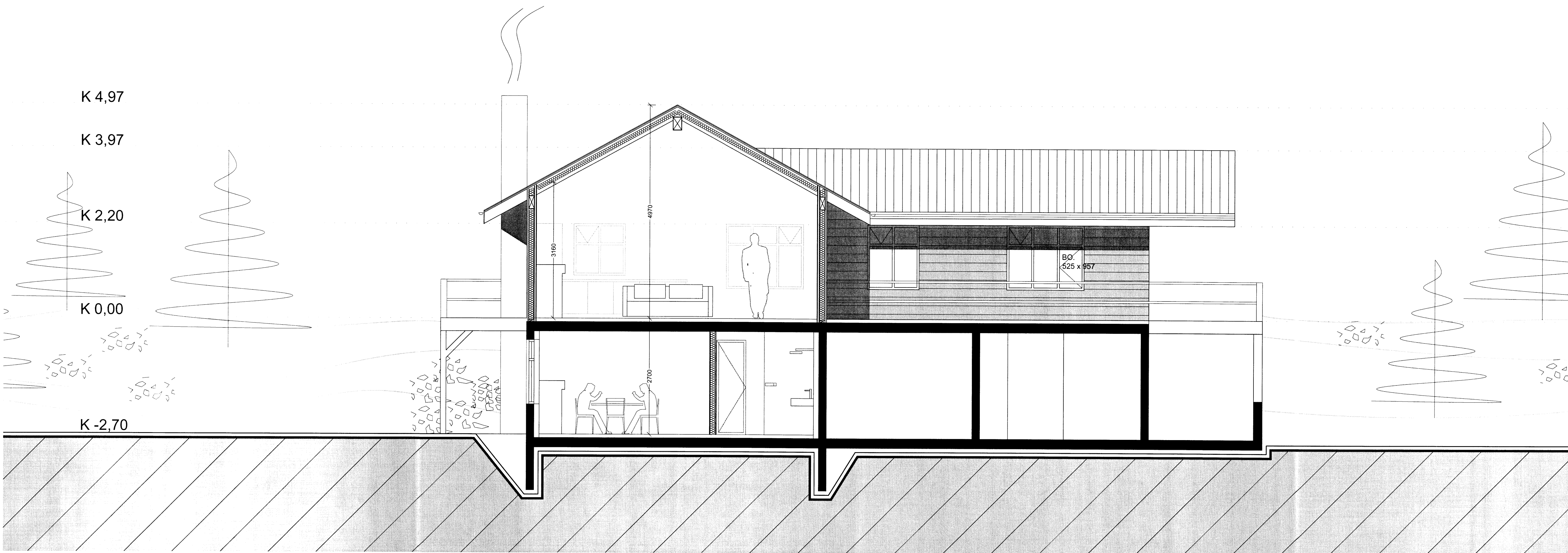
Skurður A mkv. 1:50
