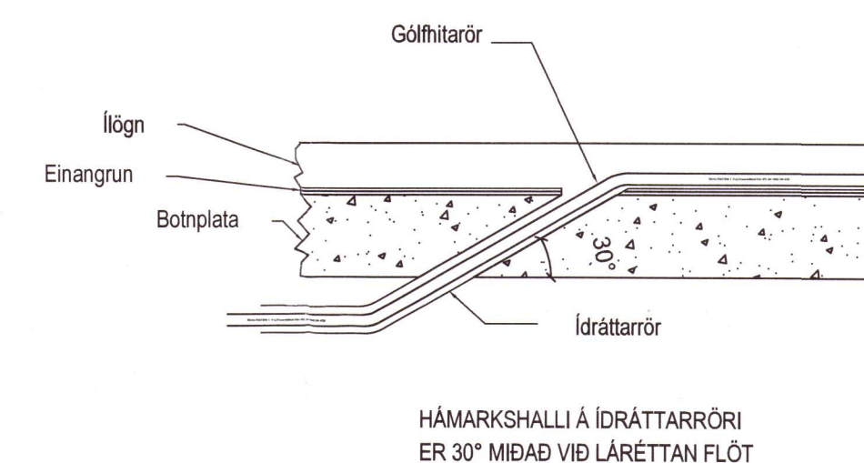
Þversnið plötu
