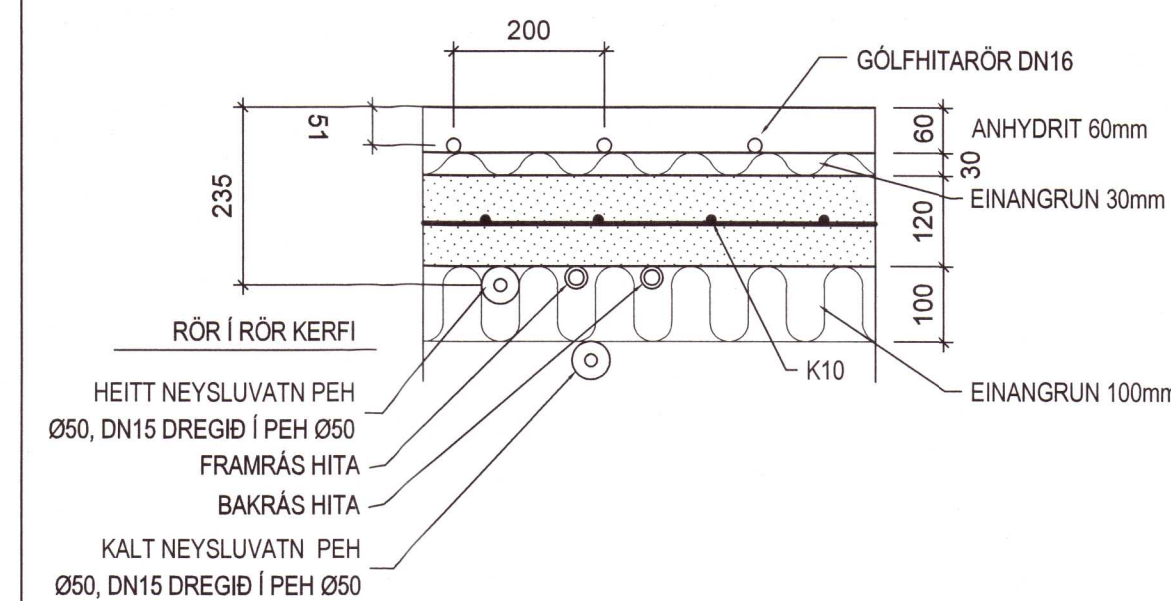
Þversnið plötu, öll mál í millimetrum
