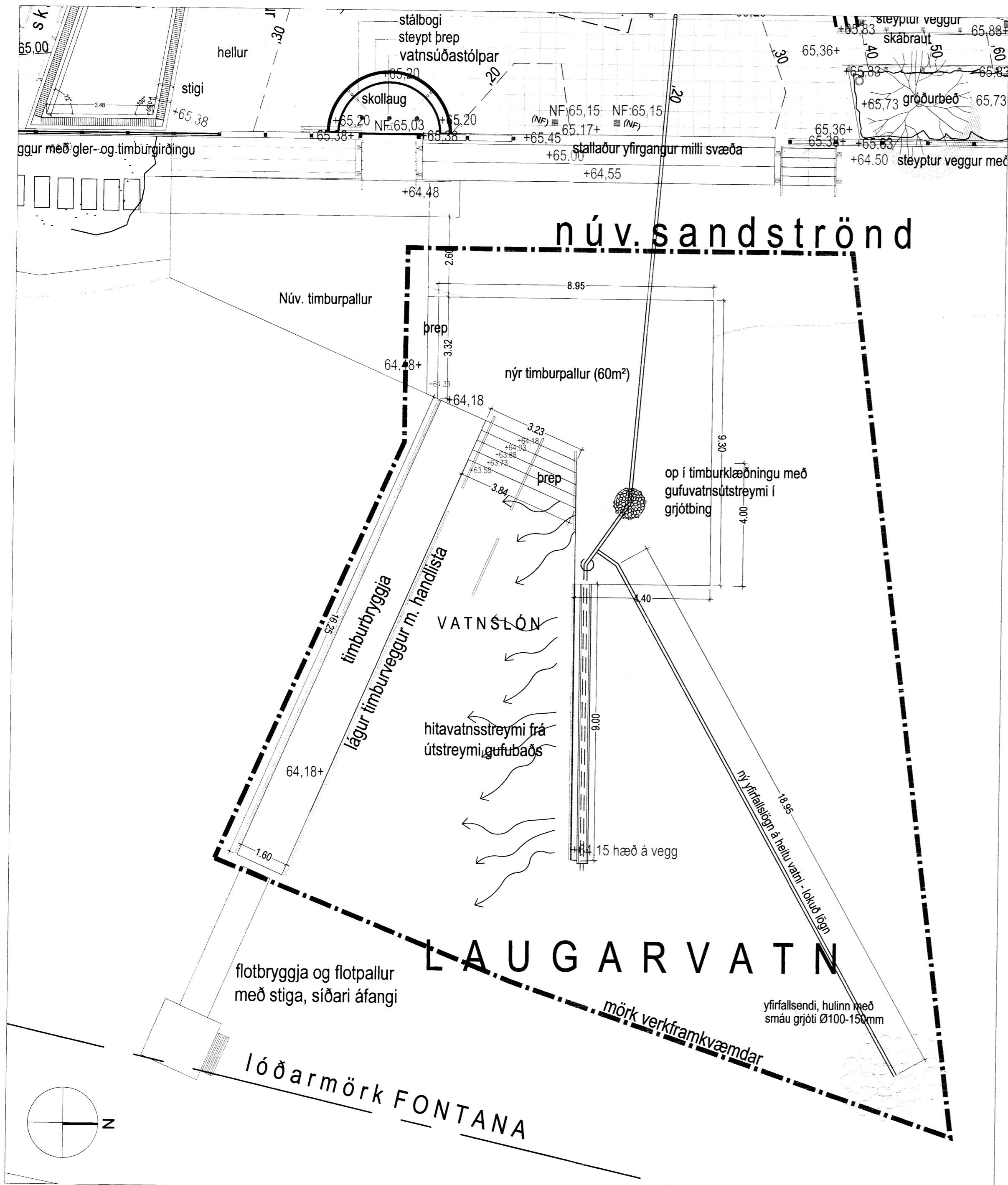
Afstöðumynd bryggju, mkv. 1:100
