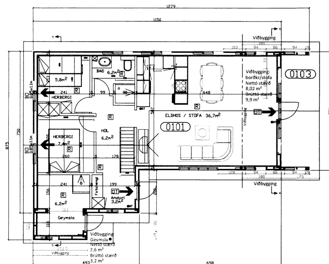
GRUNNMYND 1. HÆÐ
