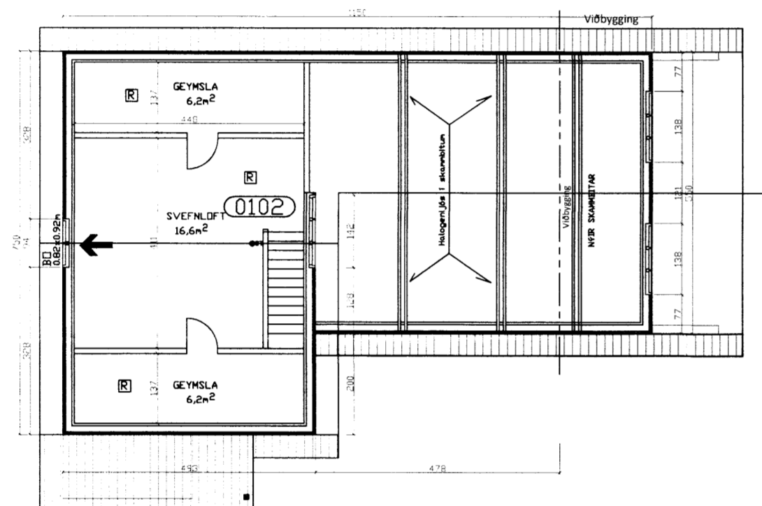
GRUNNMYND 2. HÆÐ
