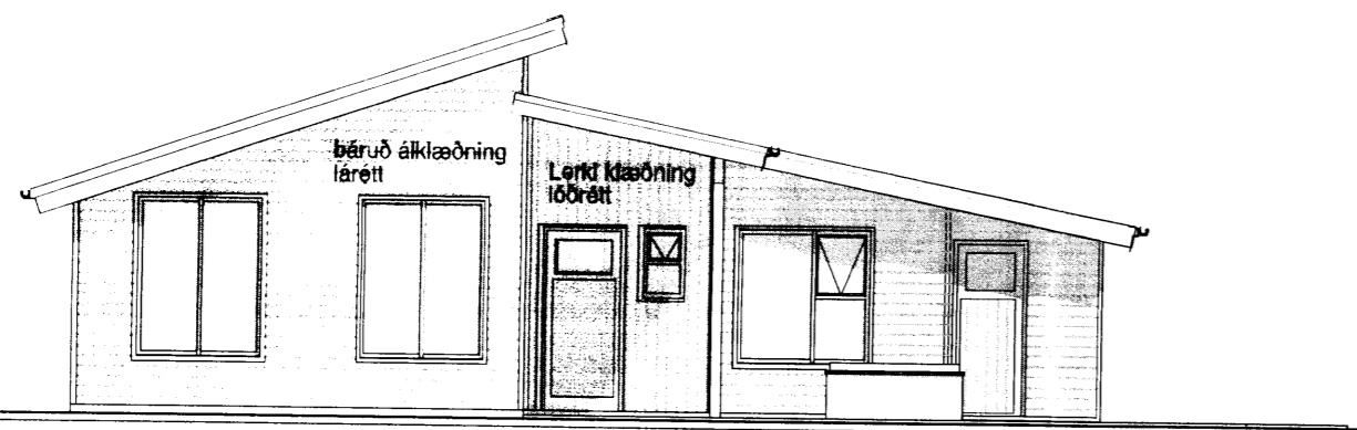
VESTUR ÚTLIT 1:100
