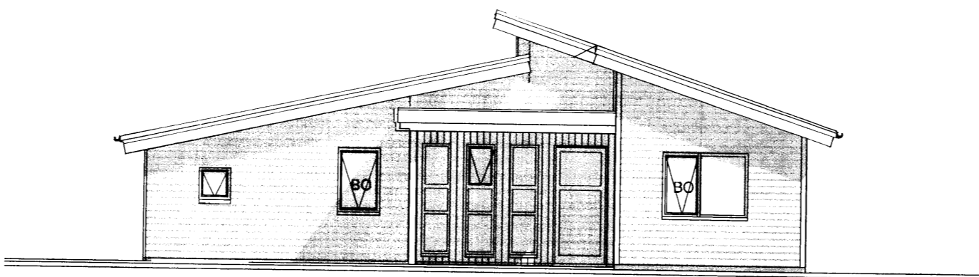
AUSTUR ÚTLIT 1:100
