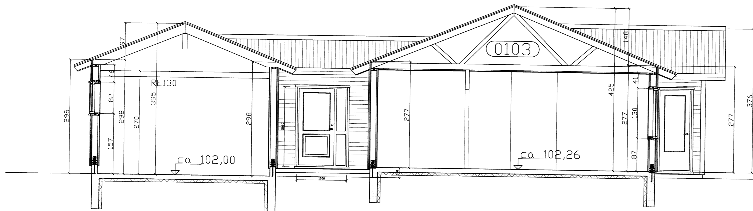
SNID A-A
