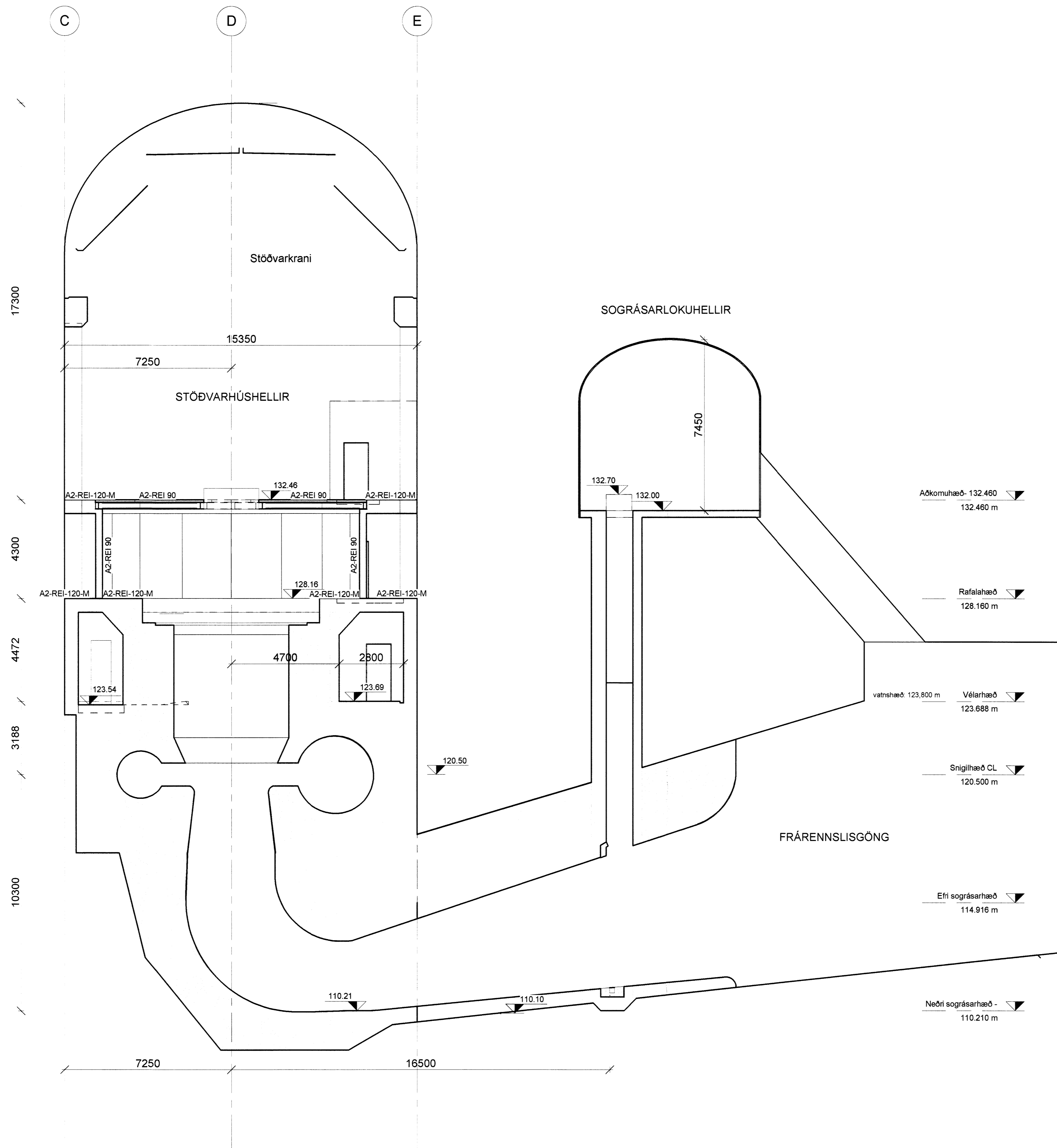
Stöðvarhús - Snið A-A 1 : 100
