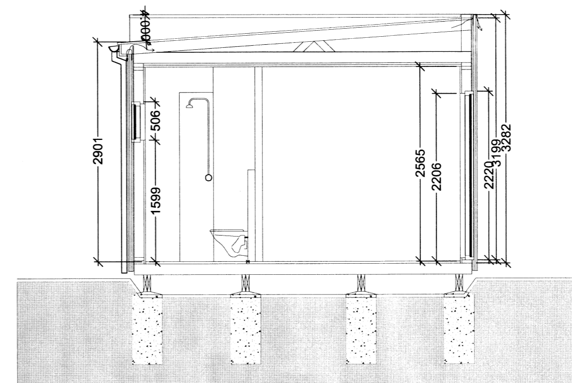
Snið í mhl. 02 M: 1:50
