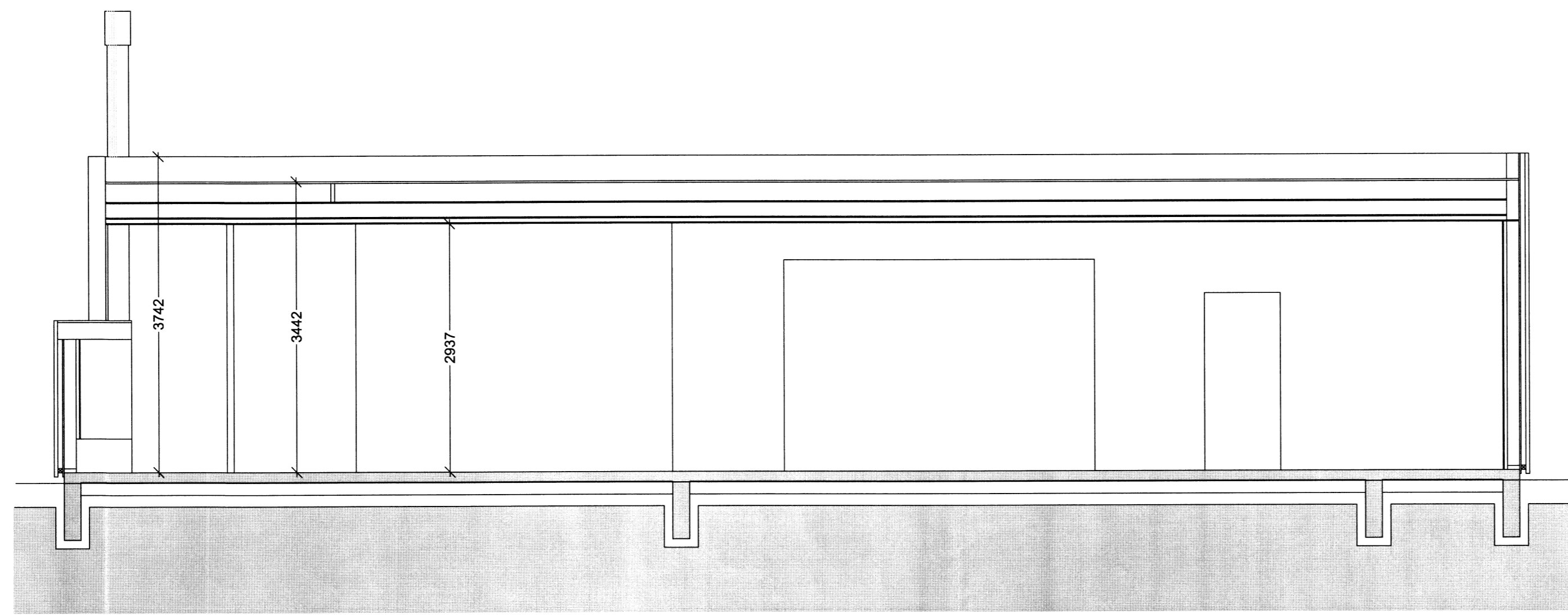
Snið í mhl. 01 M: 1:50
