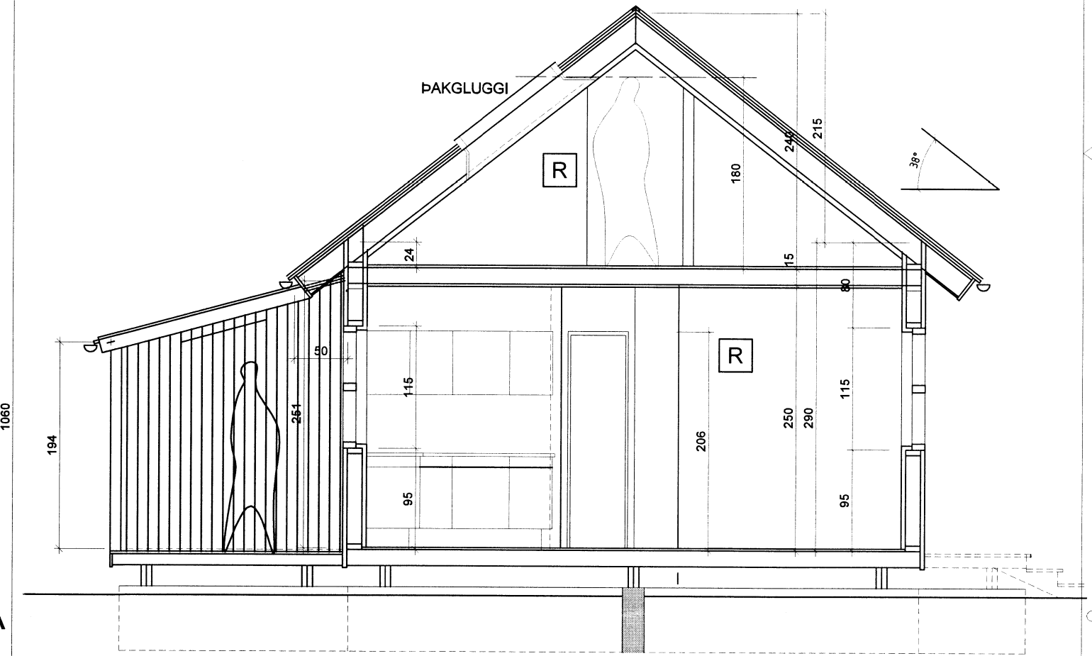
SNID A-A 1 : 50
