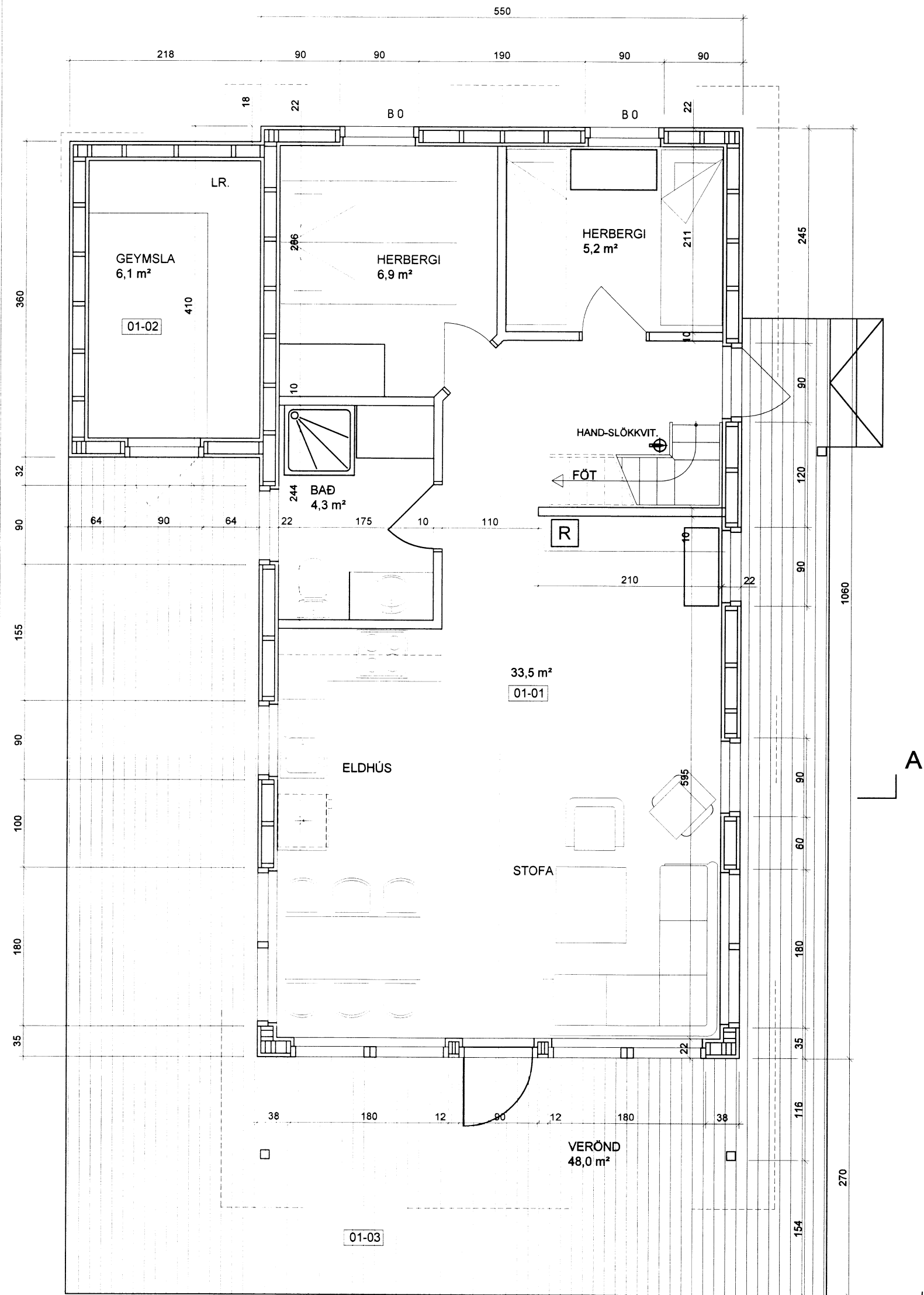
GRUNNMYND 1 : 50
