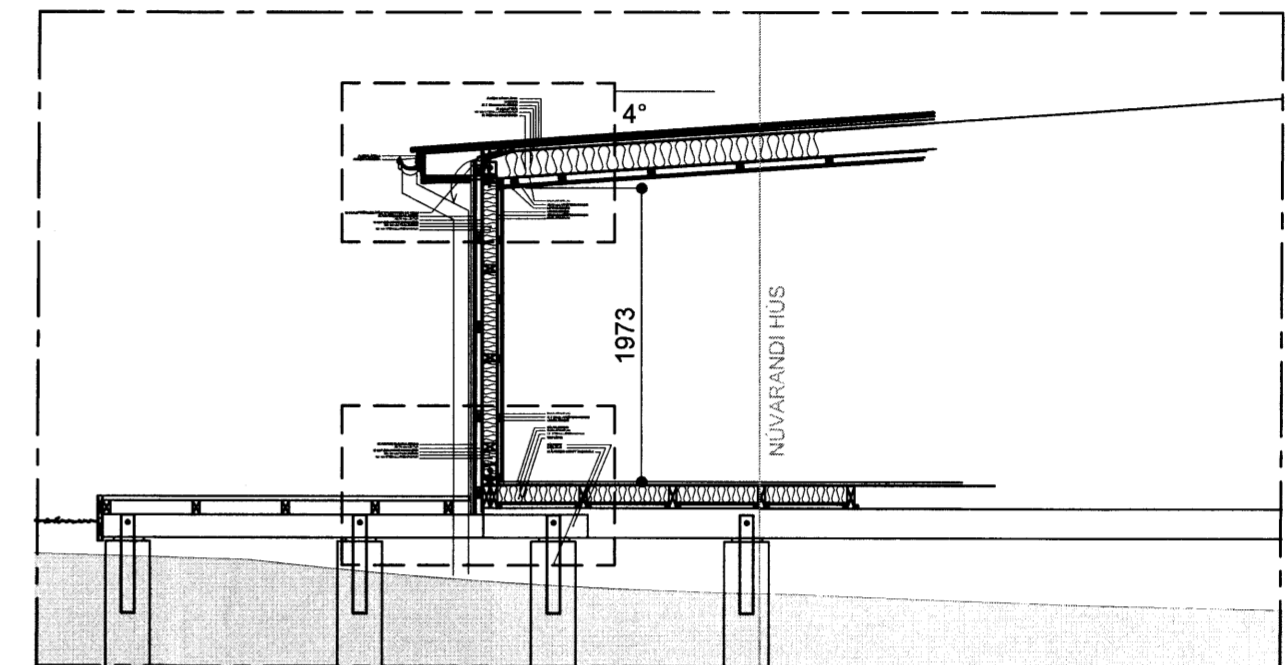
SNIÐ Í VIÐBYGGINGU MÁL 1 : 50
