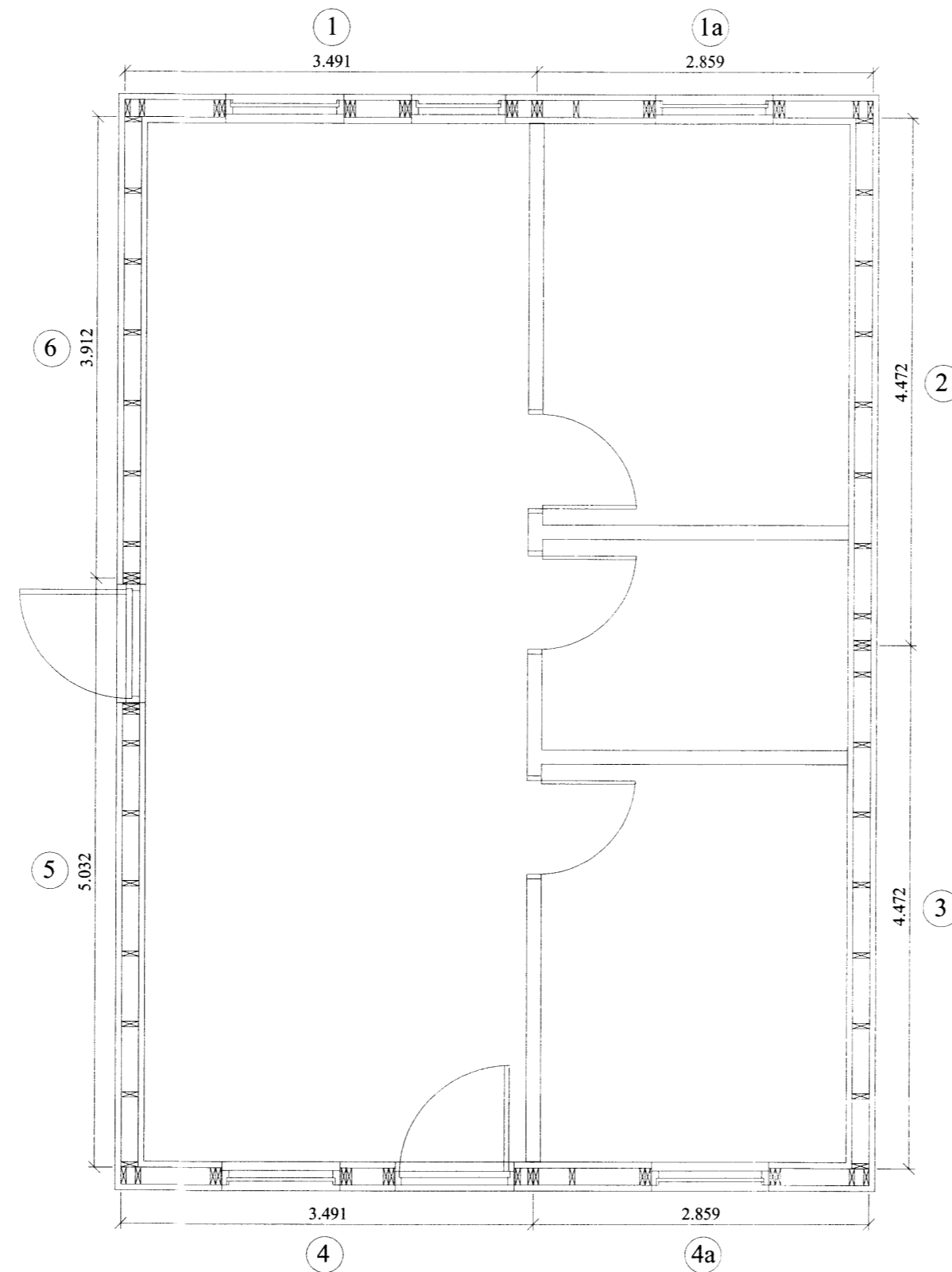
Grunnmynd grindur Mkv. 1:50
