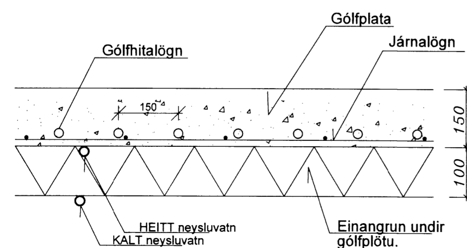
SNEIÐING, hitalagnir innsteyptar í plötu
