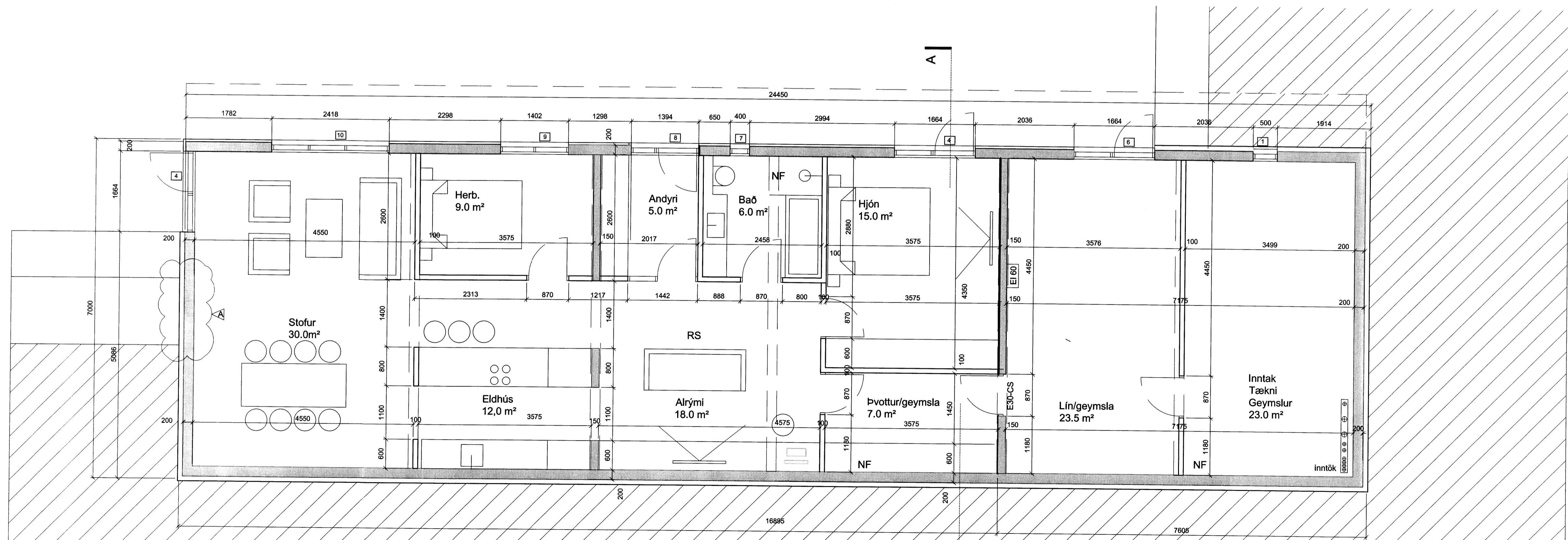
GRUNNMYND KJALLARA 1:50
