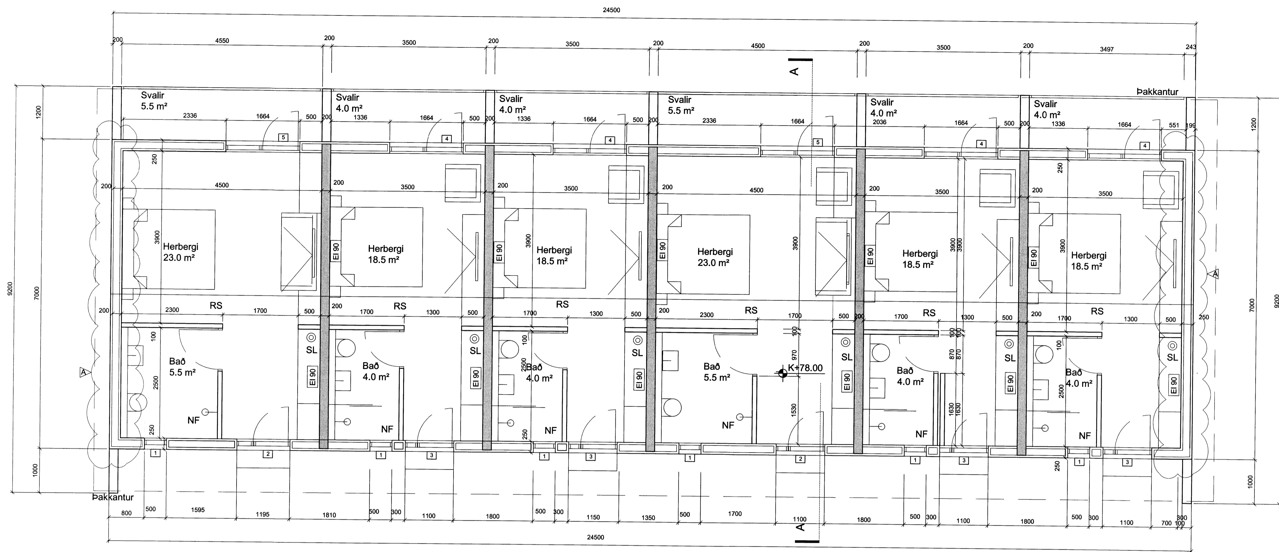
GRUNNMYND AÐALHÆÐAR 1:50
