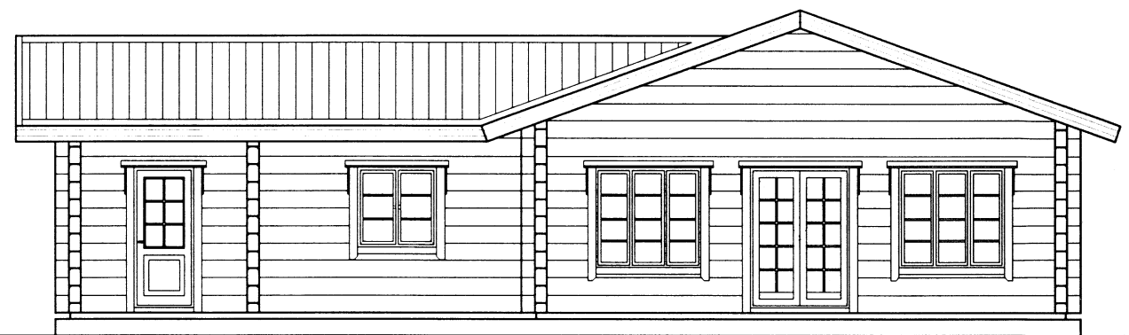
ÚTLIT SUDURHLIÐ
