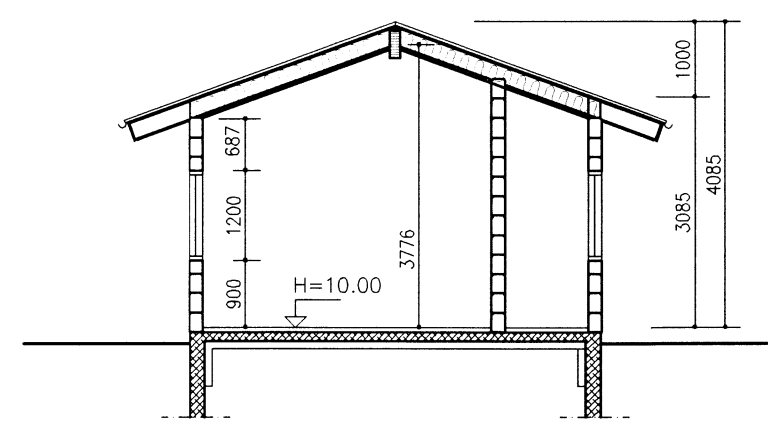
SNID 1-1 1:100
