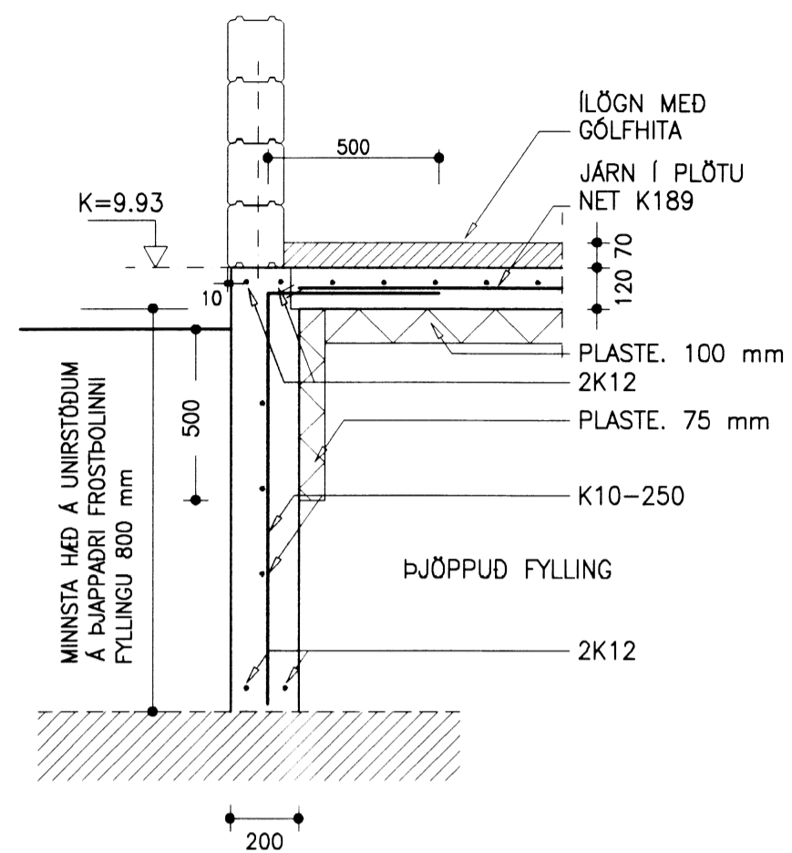
SNID 1-1 1:20
