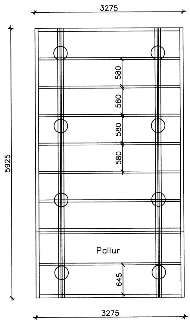
Grunnmynd dregarar
