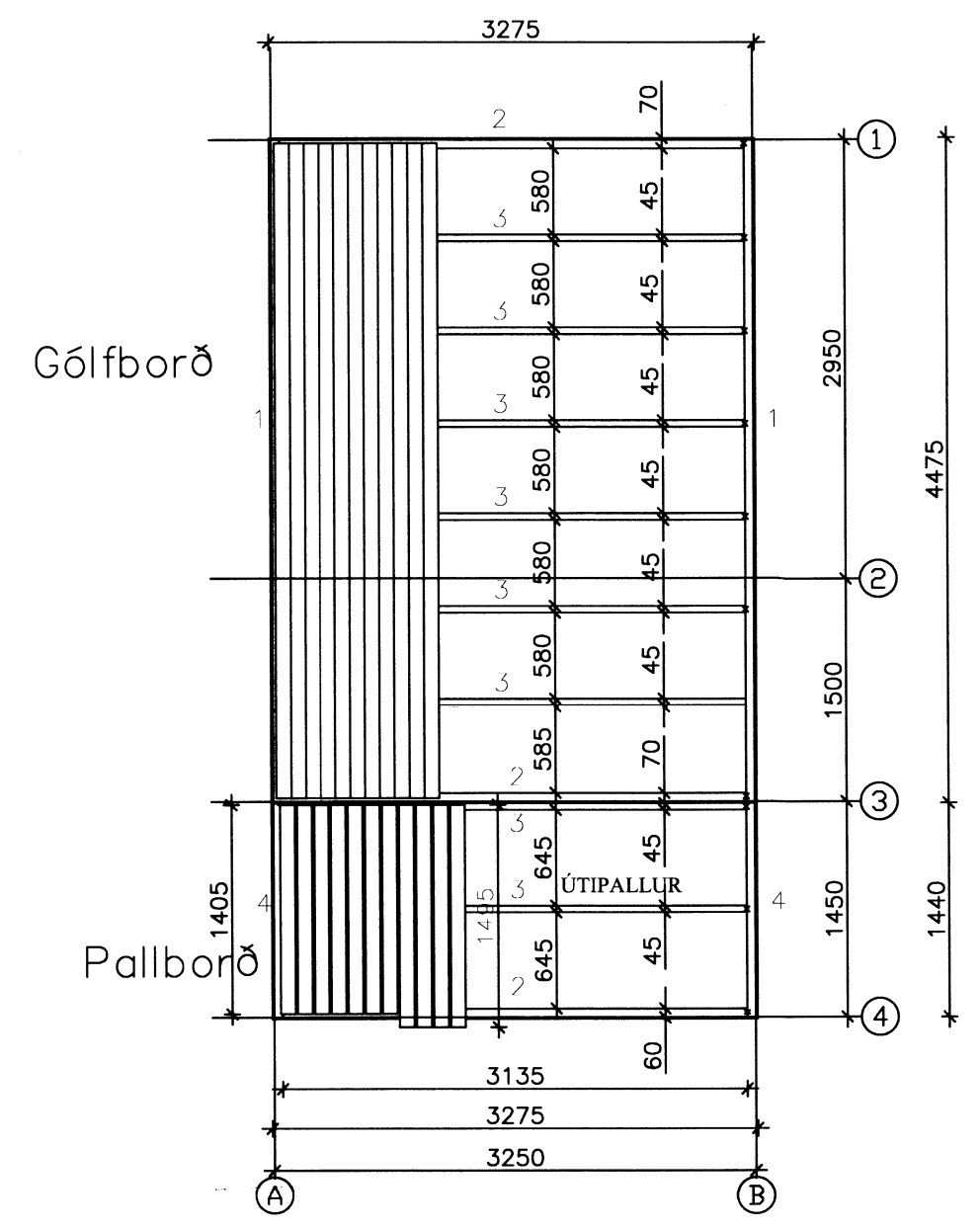
Grunnmynd gólfborð
