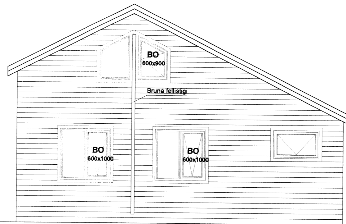
Norðurgafi eftir breytingu
